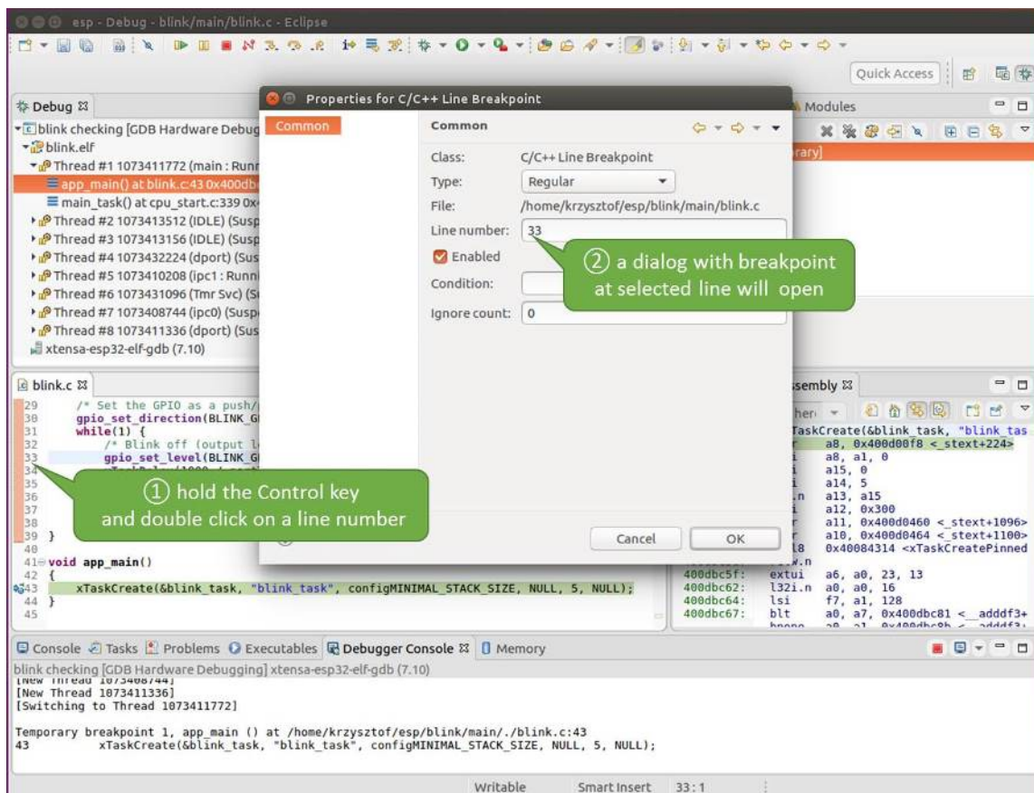
图 33: 设置断点
