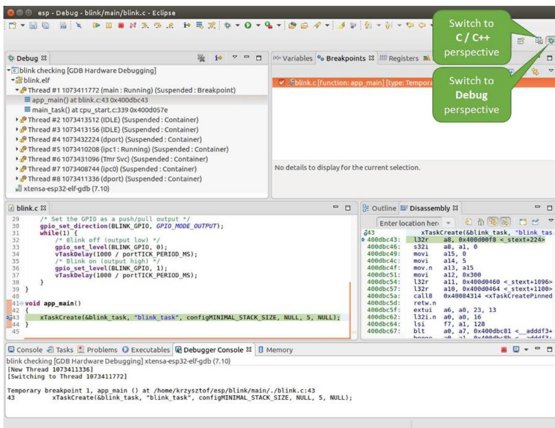
图 49: Eclipse 中的调试视图
