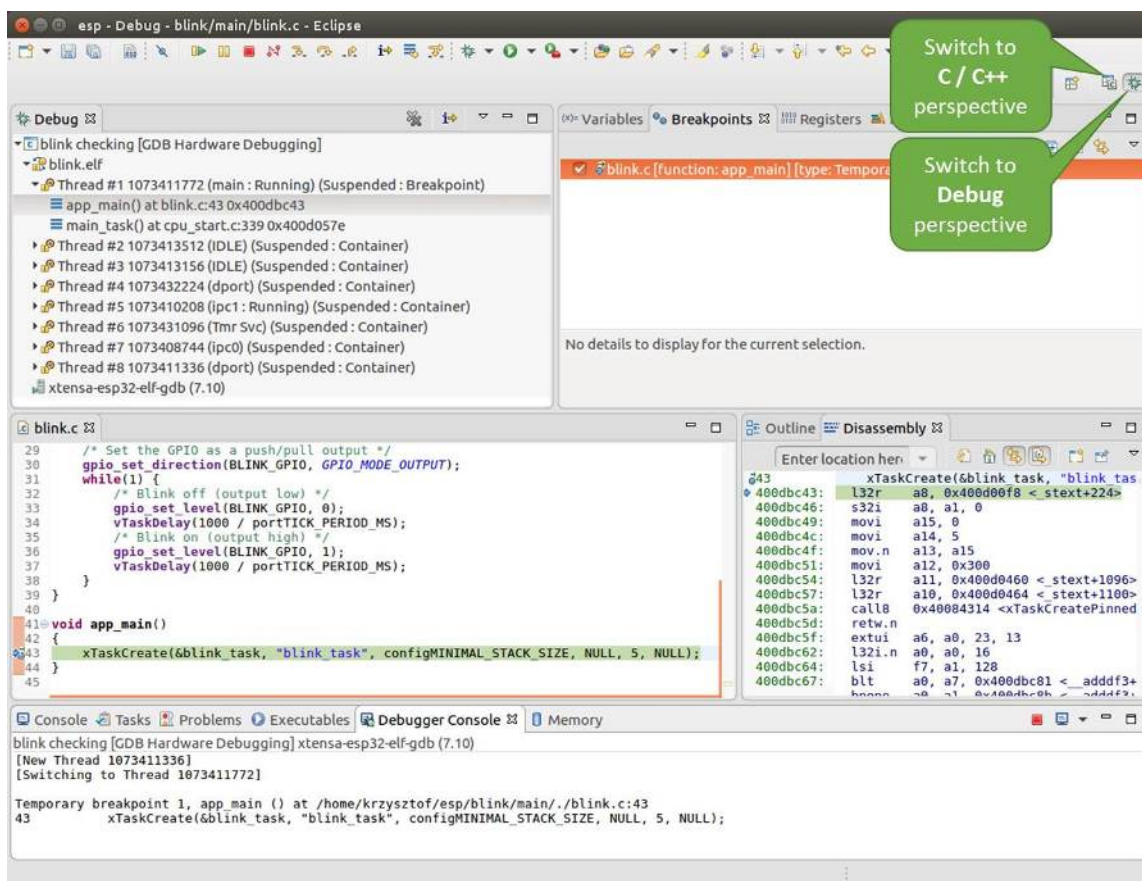
图 50: Eclipse 中的 Debug 视图
