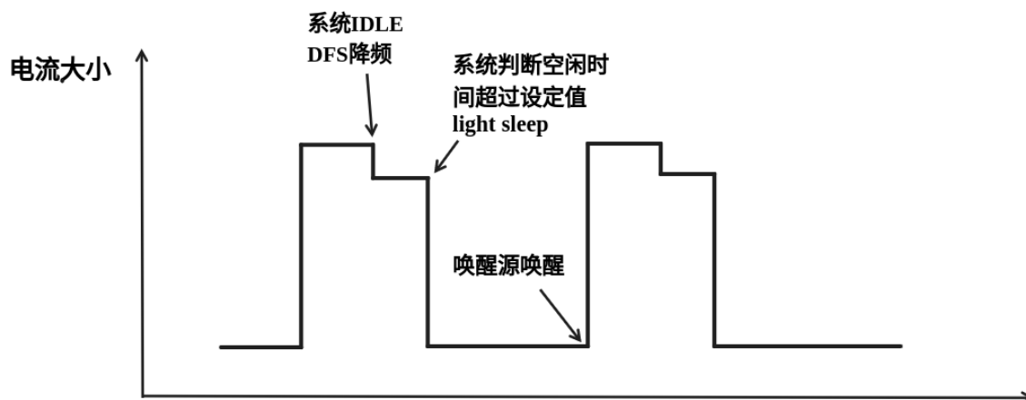
图 45: Auto Light-sleep 模式理想电流图
