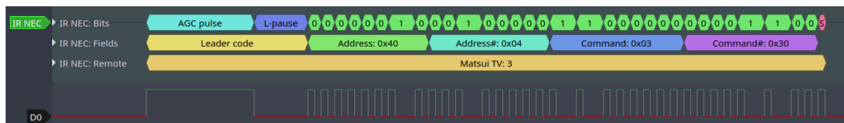
图 19: 红外 NEC 帧
