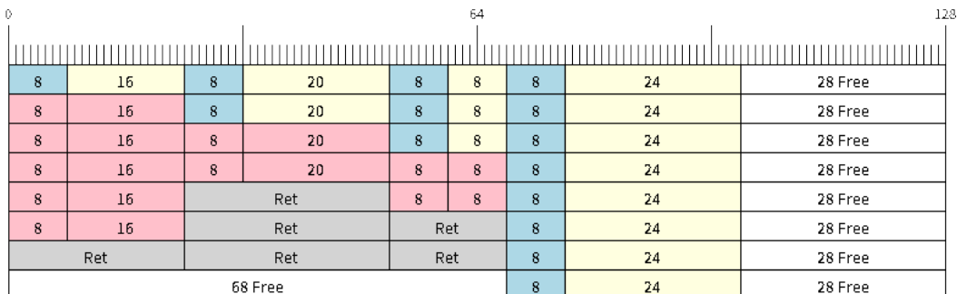
图 46: 在不可分割和可分割环形 buffer 中检索/返回数据项
