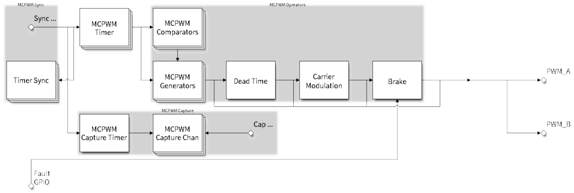
图 16: MCPWM 概述
