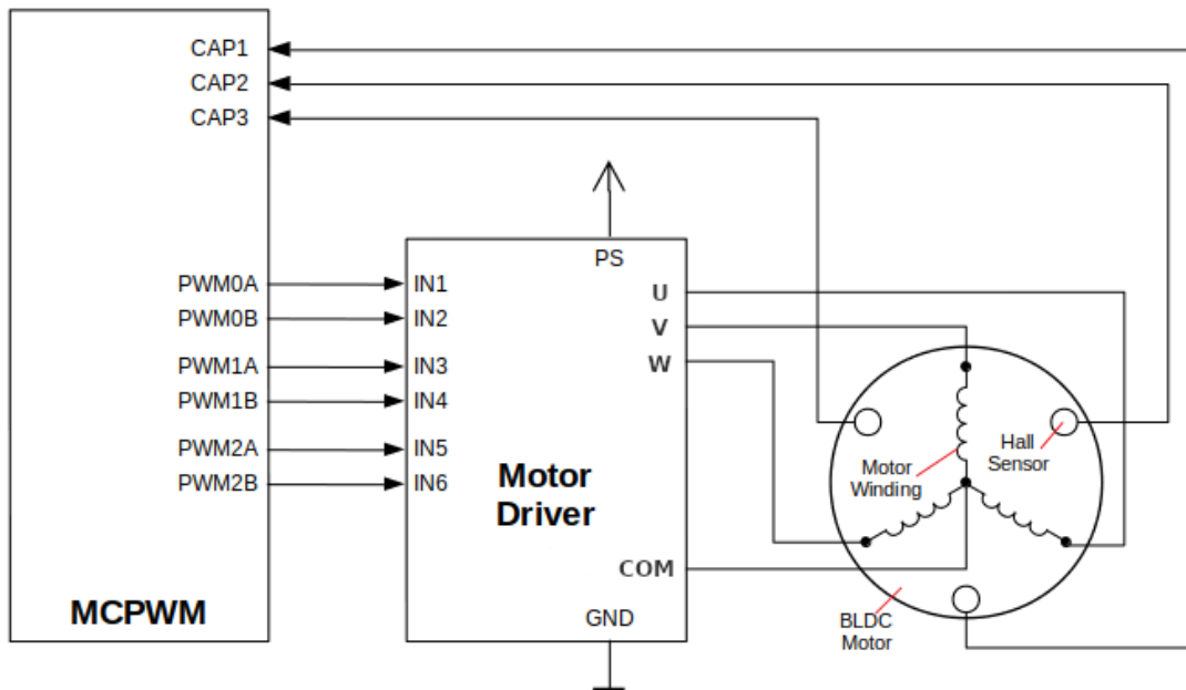
图 18: 带霍尔传感器的 MCPWM 无刷直流电机
