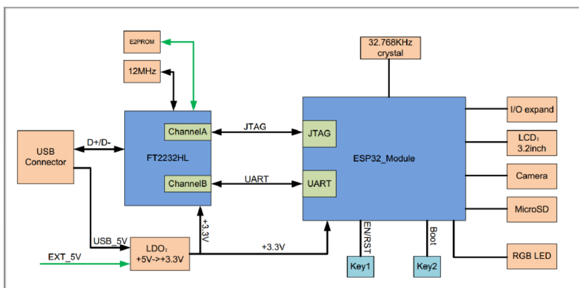
图 2: ESP-WROVER-KIT 功能框图
