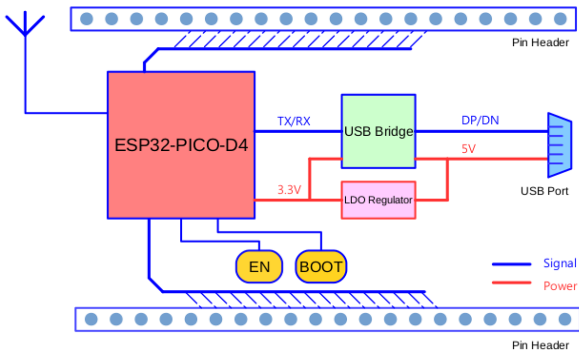
图 11: ESP32-PICO-KIT 框图
