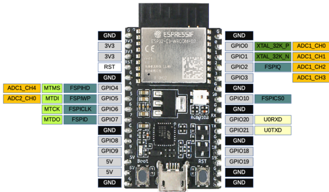
图 9: ESP32-C3-DevKitC-02 管脚布局
