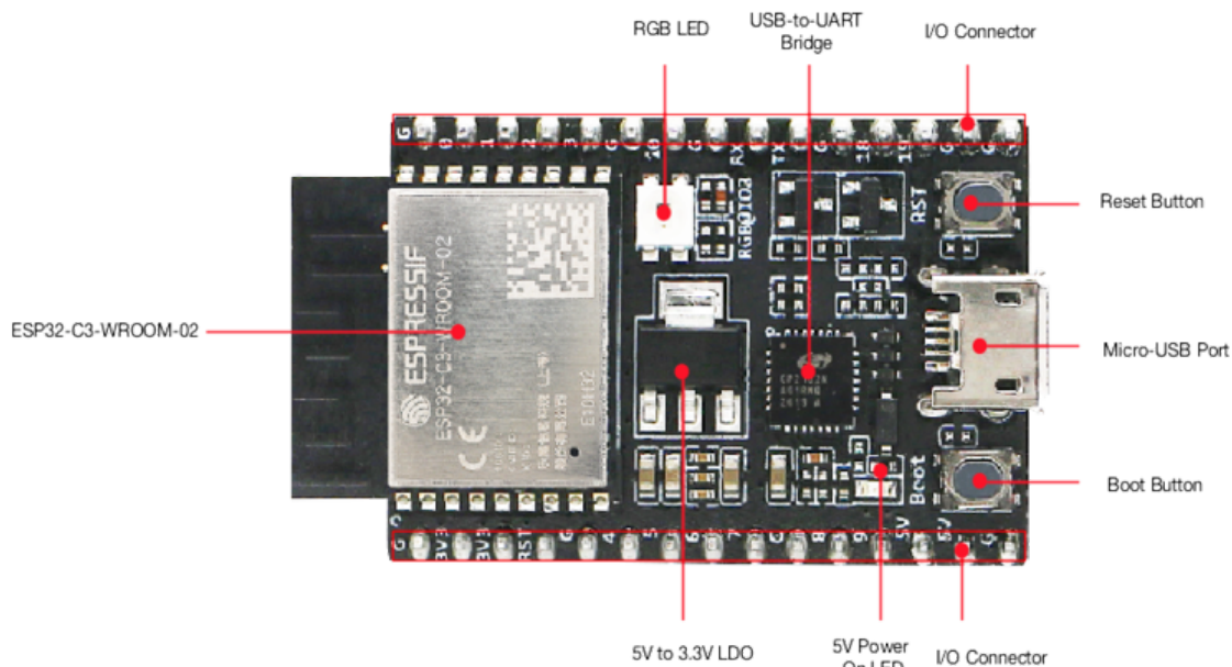
图 7: ESP32-C3-DevKitC-02 - 正面
