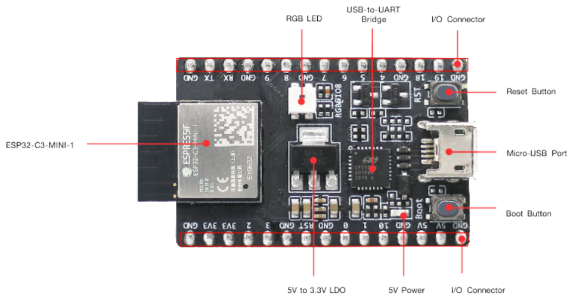
图 3: ESP32-C3-DevKitM-1 - 正面
