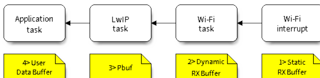
图 61: 接收数据缓冲区分配
