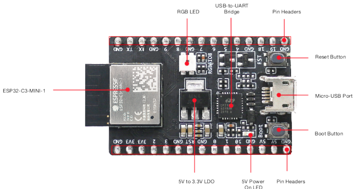
图 3: ESP32-C3-DevKitM-1 - 正面
