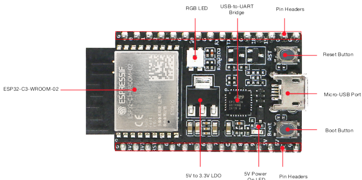
图 7: ESP32-C3-DevKitC-02 - 正面
