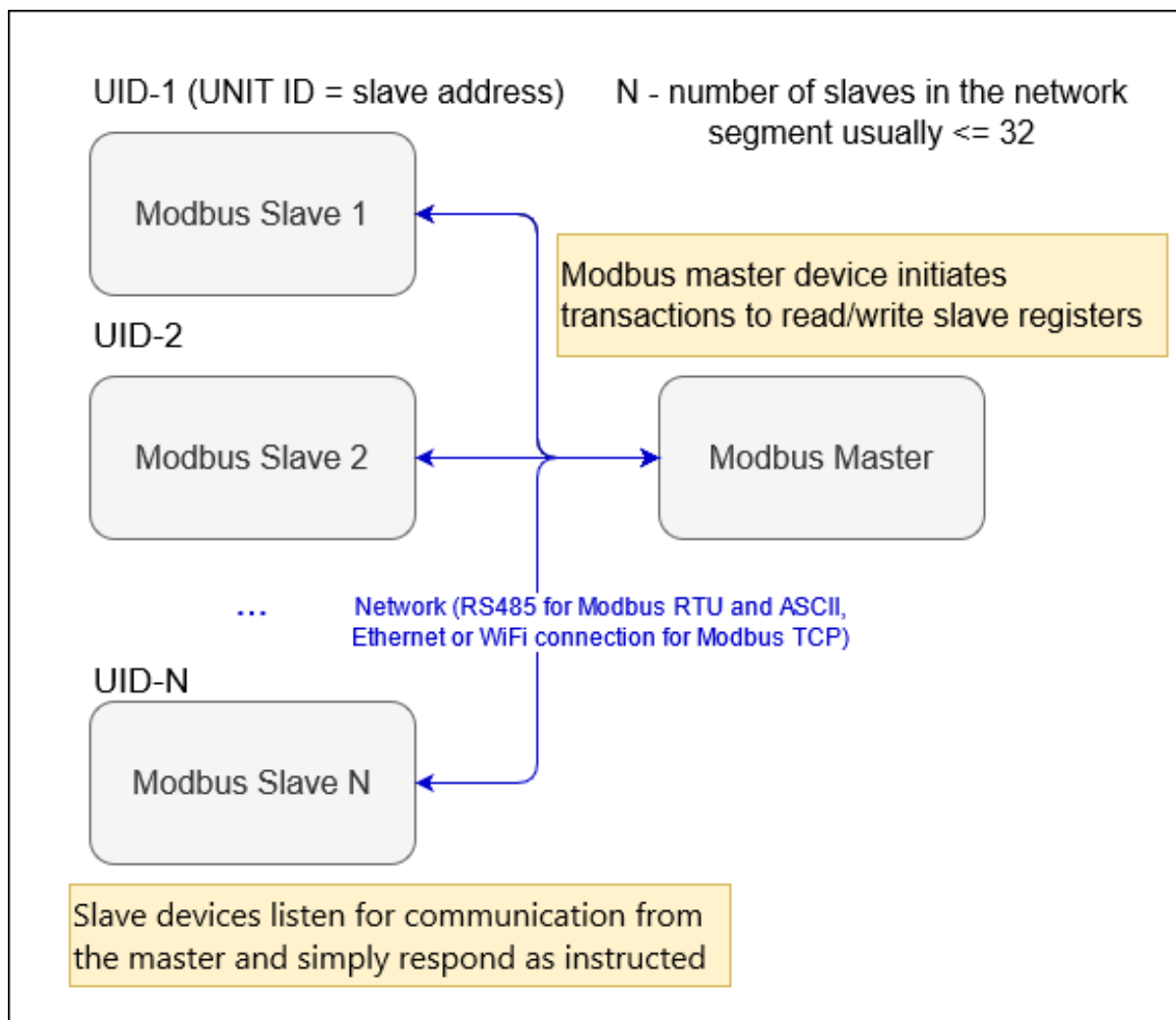
图 16: Modbus segment diagram
