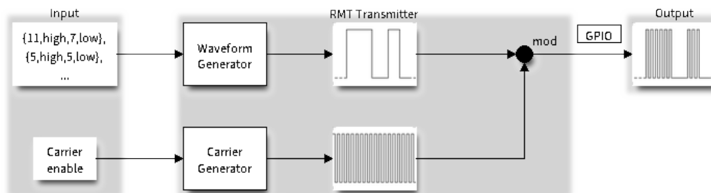
图 7: RMT Transmitter Overview
