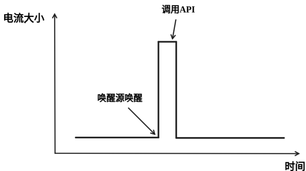
图 64: Deep-sleep 模式理想电流图
