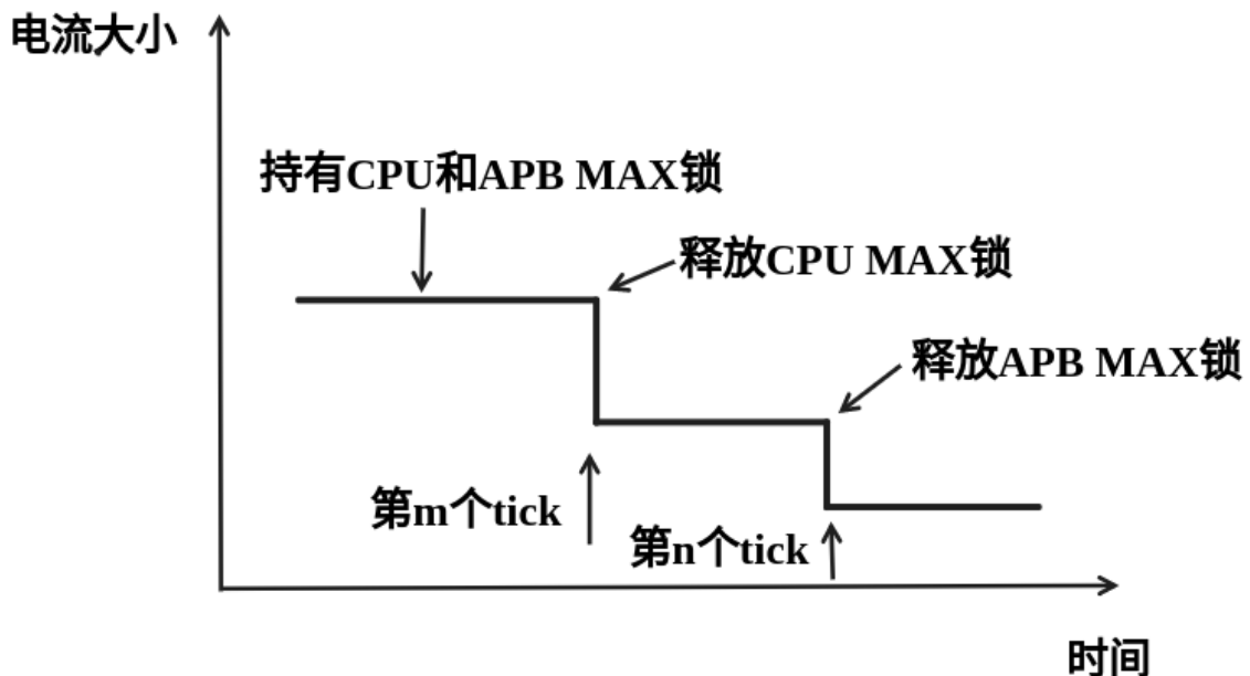
图 60: 理想 DFS 机制调频电流图
