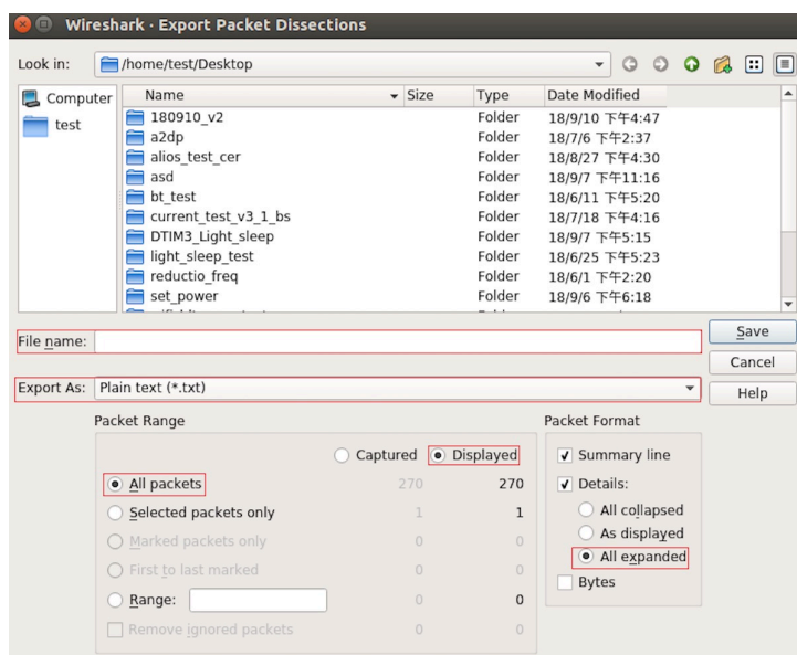
图 83: 保存捕捉包
