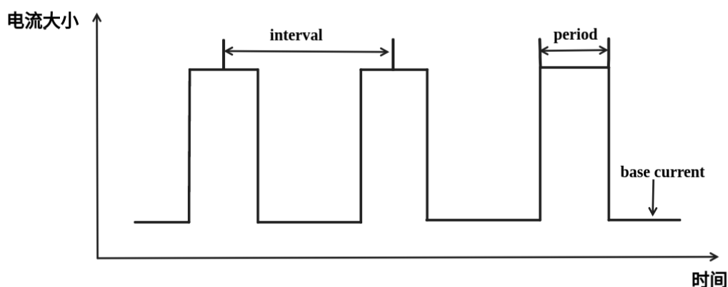
图 67: 理想情况下 WiFi 场景低功耗模式电流图
