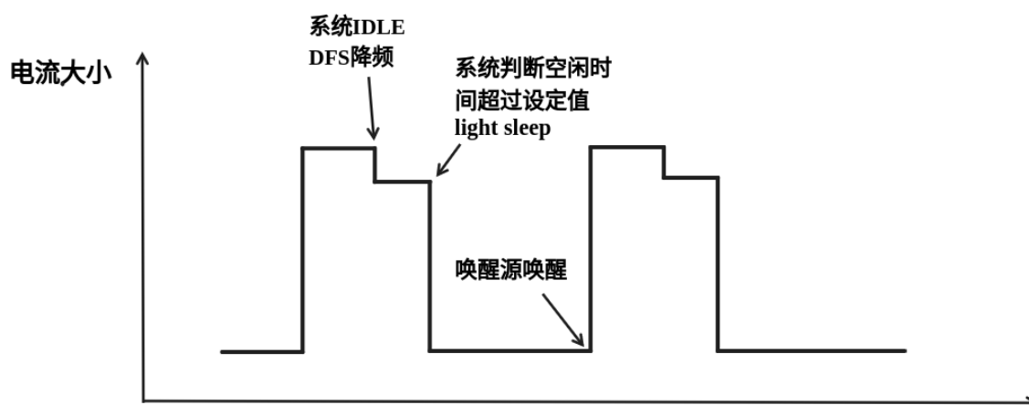
图 62: Auto Light-sleep 模式理想电流图
