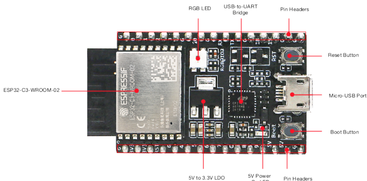
图 7: ESP32-C3-DevKitC-02 - 正面
