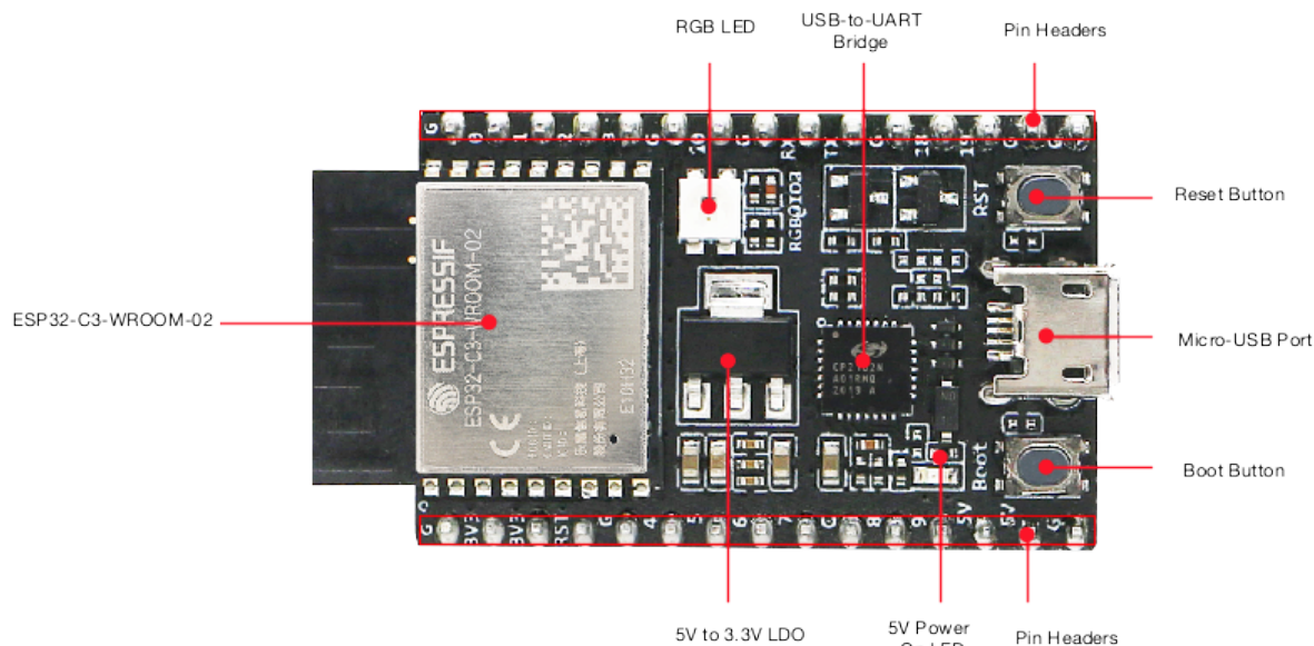
图 7: ESP32-C3-DevKitC-02 - 正面
