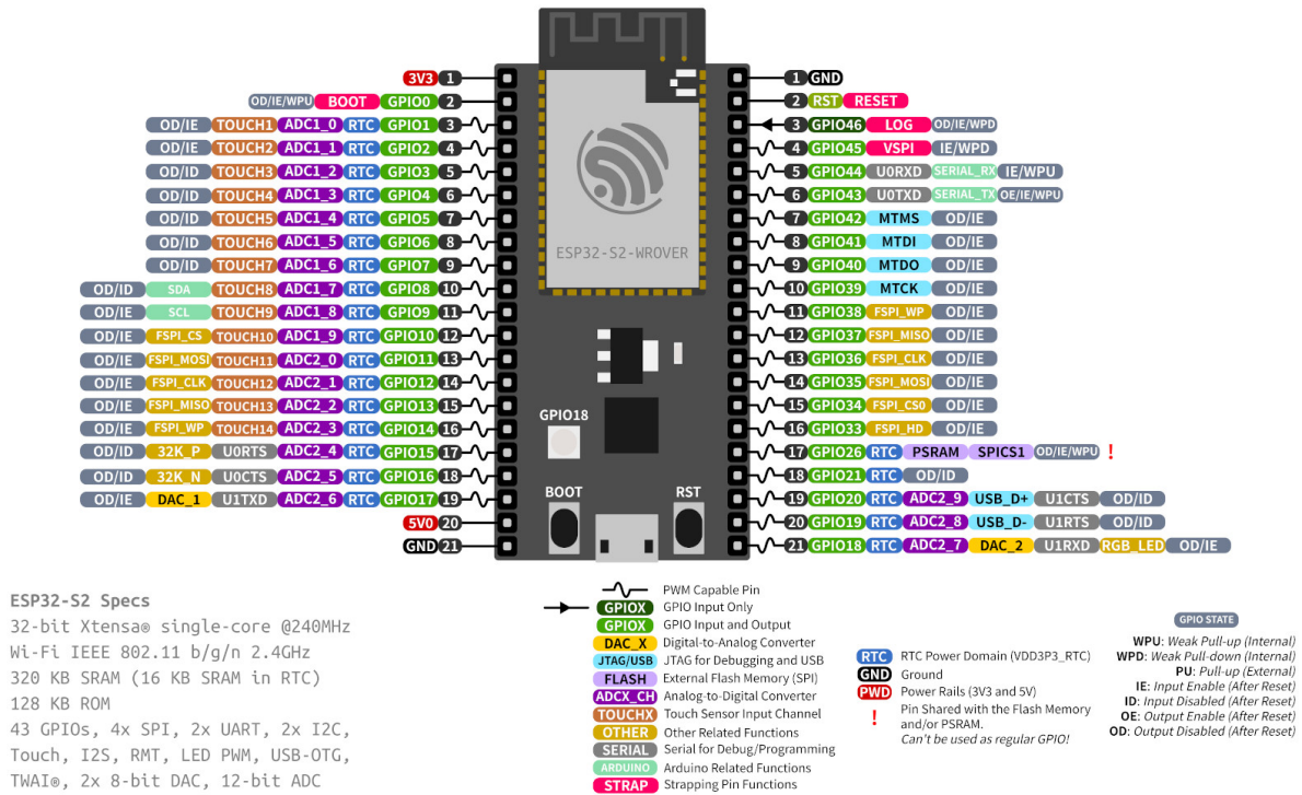
图 5: ESP32-S2-Saola-1 管脚布局 (点击放大)
