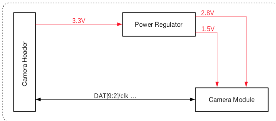
图 34: ESP-LyraP-CAM 功能框图
