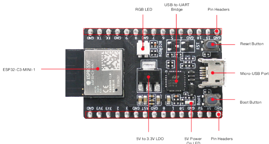
图 2: ESP32-C3-DevKitM-1 - 正面
