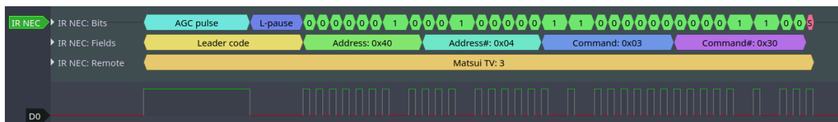
图 15: 红外 NEC 帧
