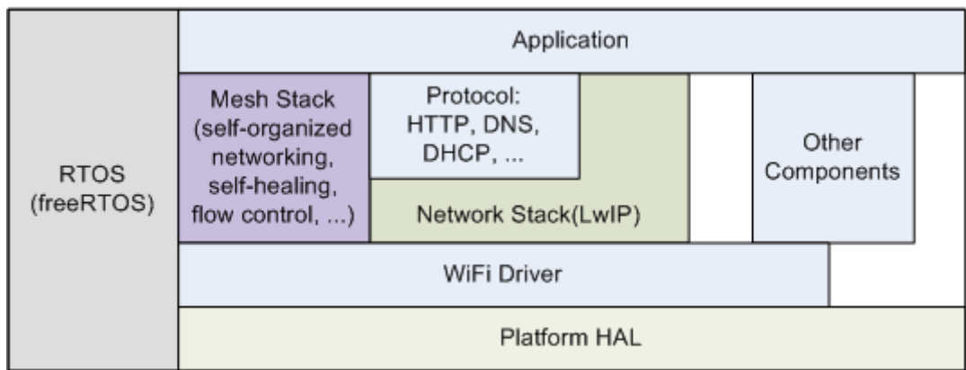
图 2: ESP-WIFI-MESH 软件栈
