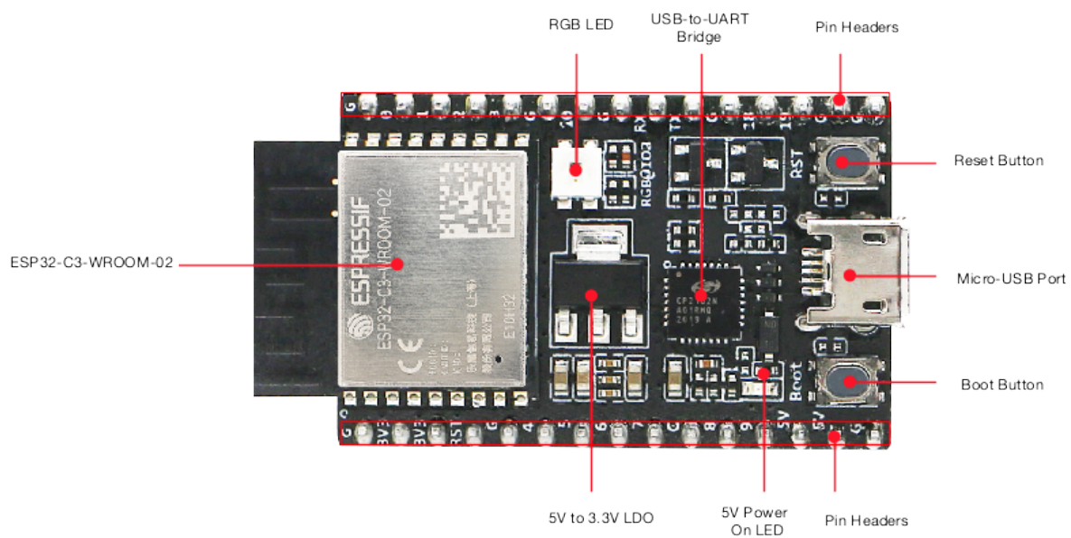
图 6: ESP32-C3-DevKitC-02 - 正面
