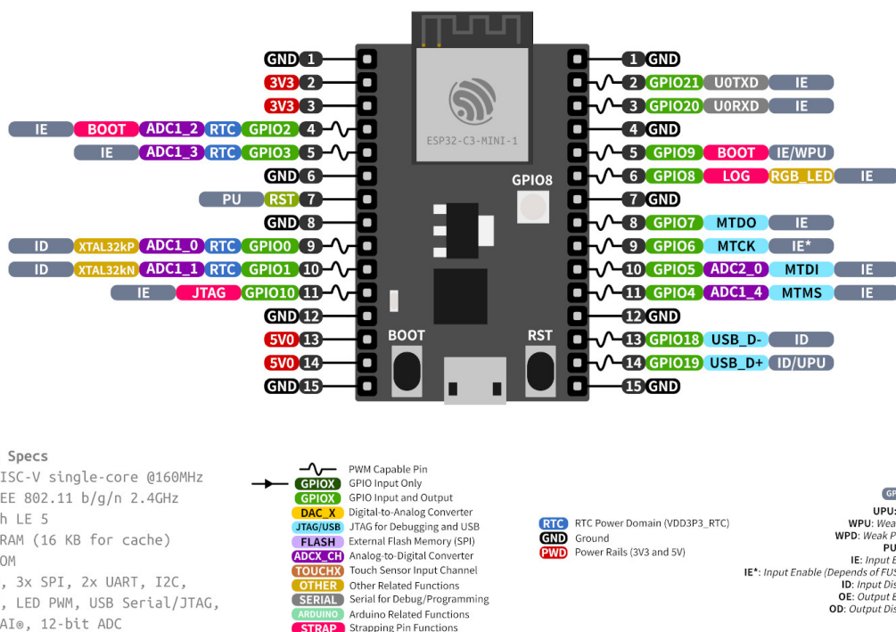
图 4: ESP32-C3-DevKitM-1 管脚布局 (点击放大)
