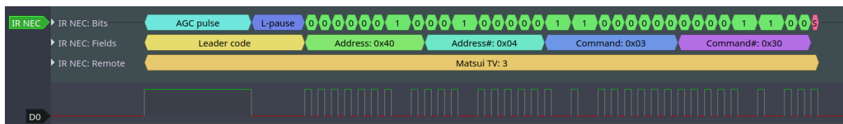
图 15: 红外 NEC 帧
