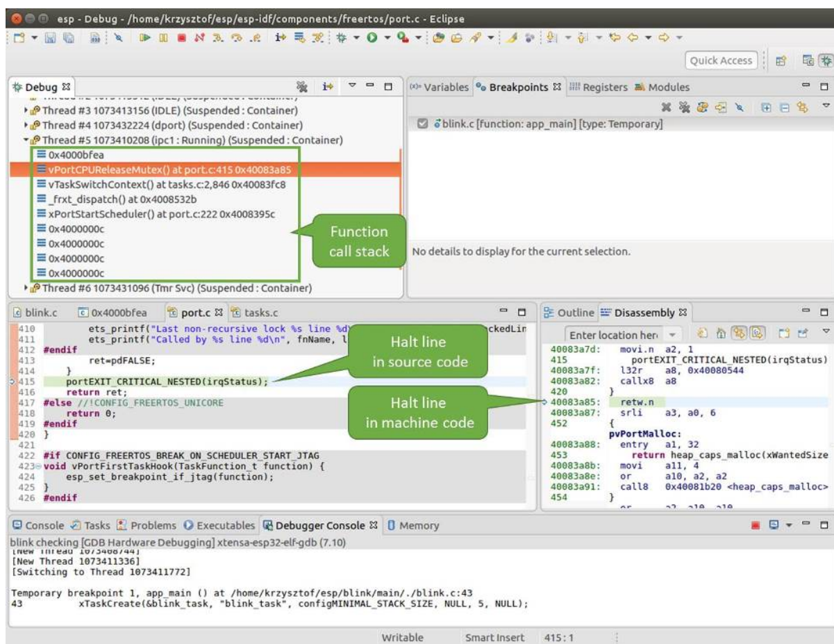
图 15: 浏览函数调用堆栈
