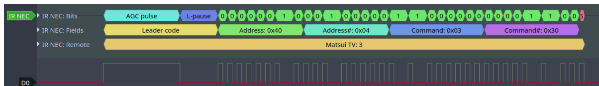
图 18: 红外 NEC 帧
