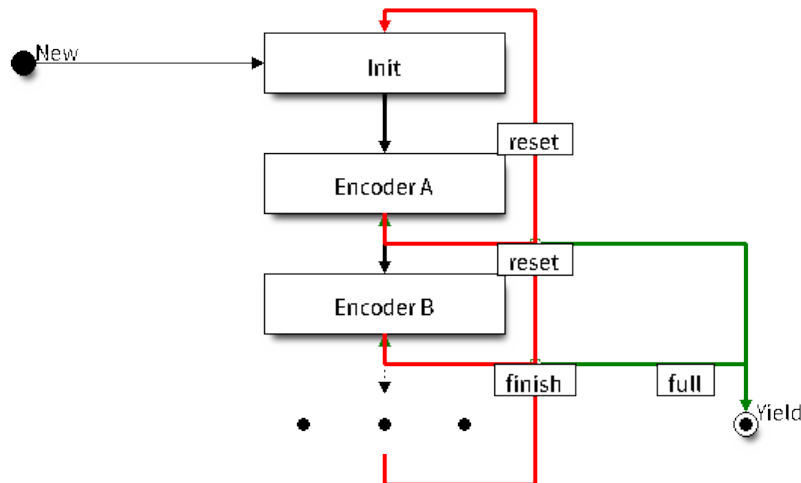
图 16: RMT Encoder Chain
