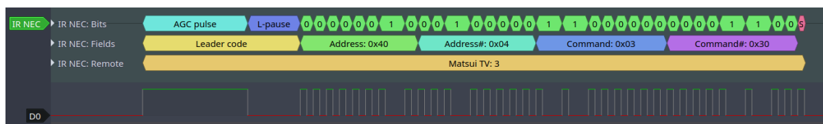
图 17: IR NEC Frame
