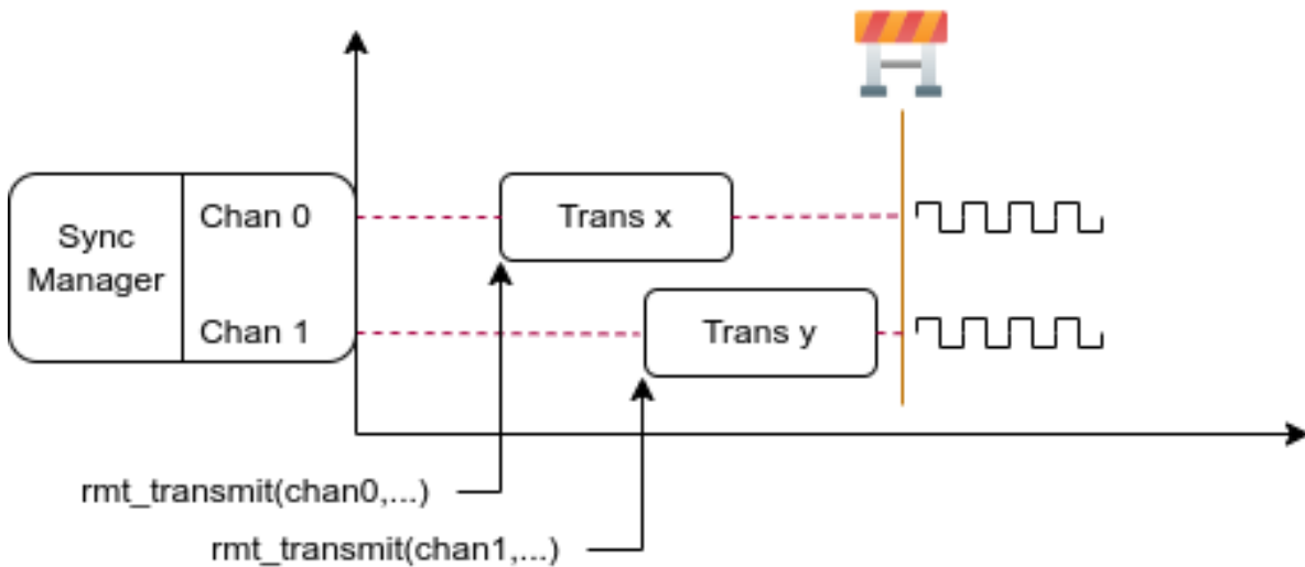
图 15: RMT TX Sync
