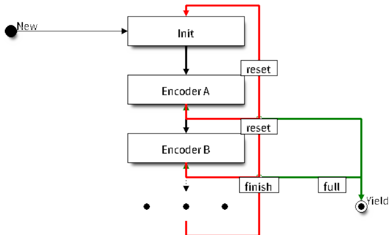
图 18: RMT Encoder Chain
