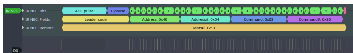
图 15: IR NEC Frame
