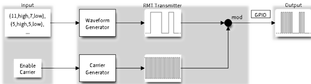
图 11: RMT 发射器概述
