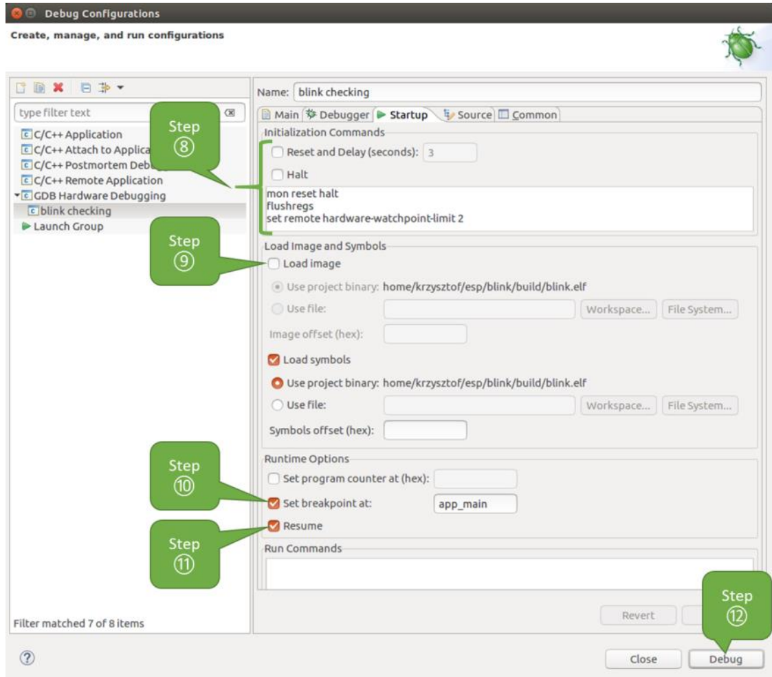
图 22: GDB 硬件调试的配置 - Startup 选项卡
