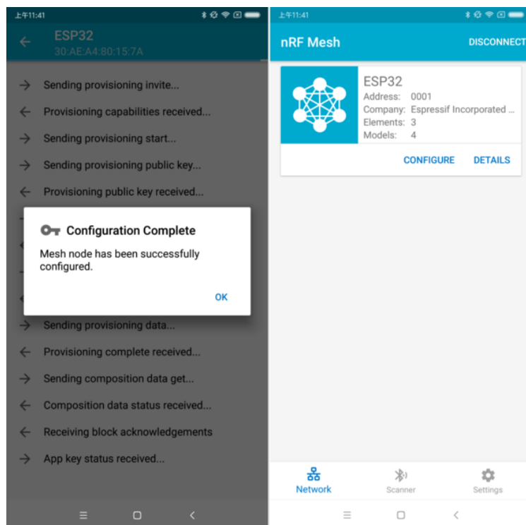
图 9: nRF Mesh - 配置完成
