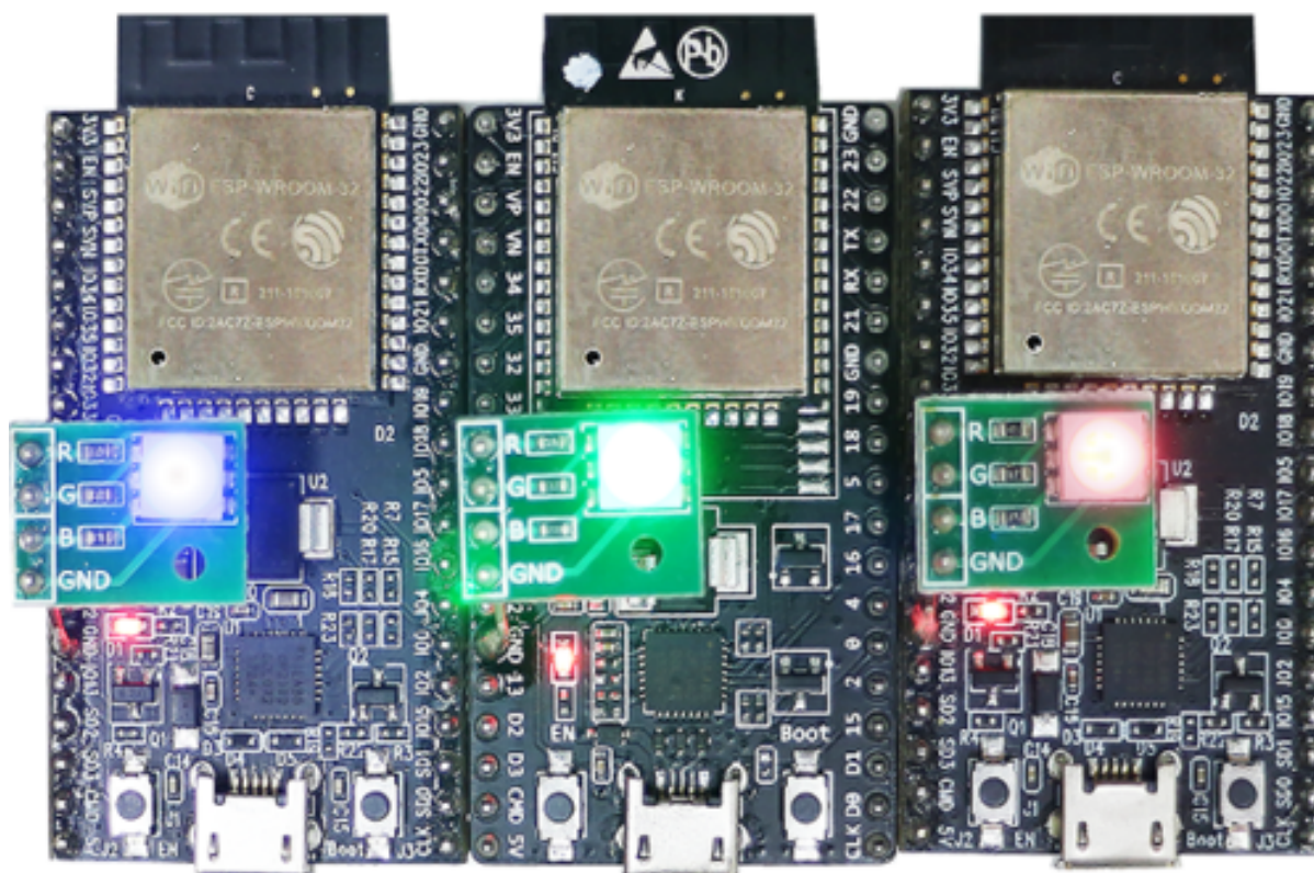
图 15: 3 个上电的 ESP-BLE-MESH 节点
