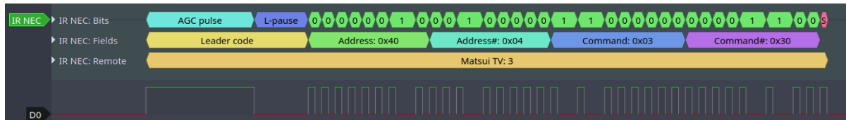
图 17: 红外 NEC 帧
