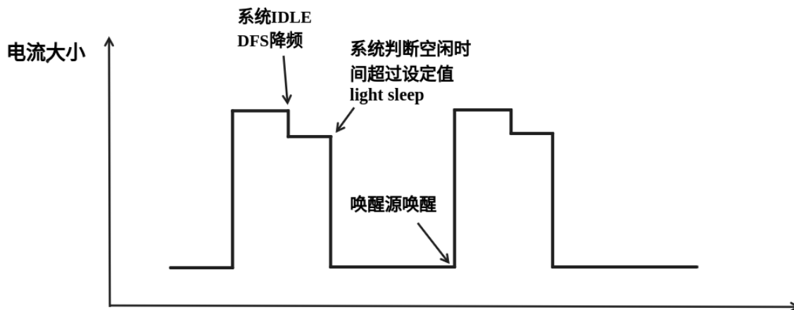
图 67: Auto Light-sleep 模式理想电流图
