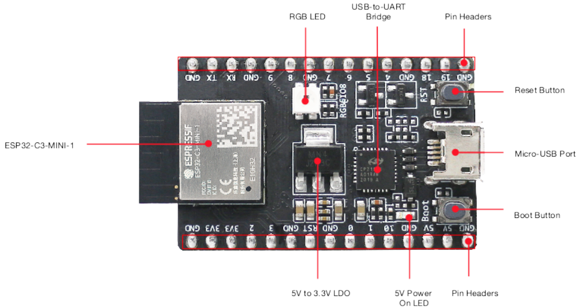
图 2: ESP32-C3-DevKitM-1 - 正面
