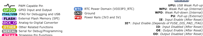
图 4: ESP32-C3-DevKitM-1 管脚布局 (点击放大)
