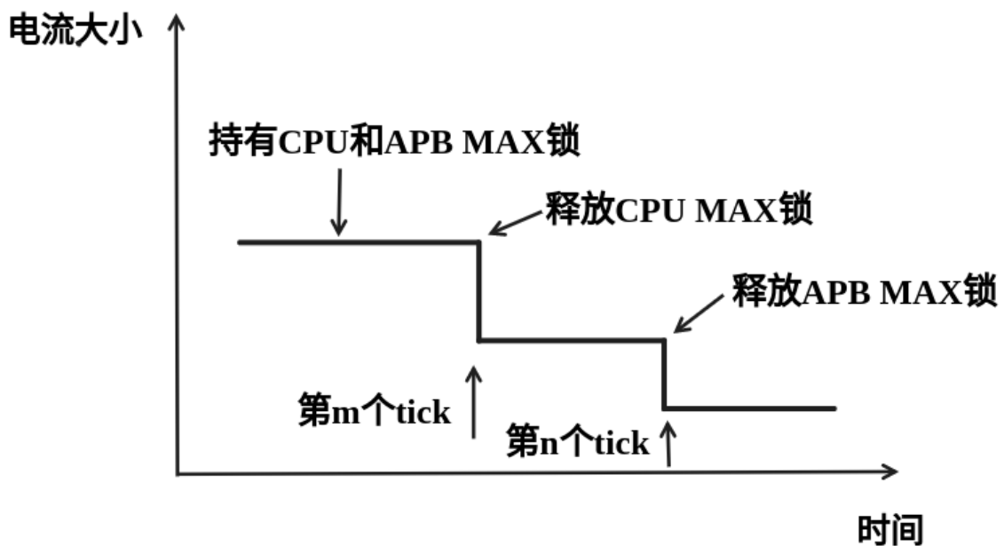
图 37: 理想 DFS 机制调频电流图
