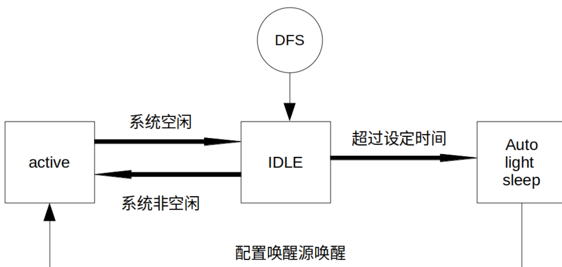
图 38: Auto Light-sleep 模式工作流程图
