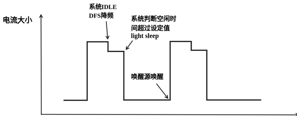
图 39: Auto Light-sleep 模式理想电流图
