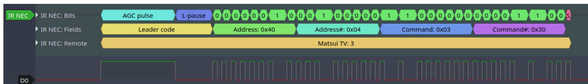
图 17: 红外 NEC 帧
