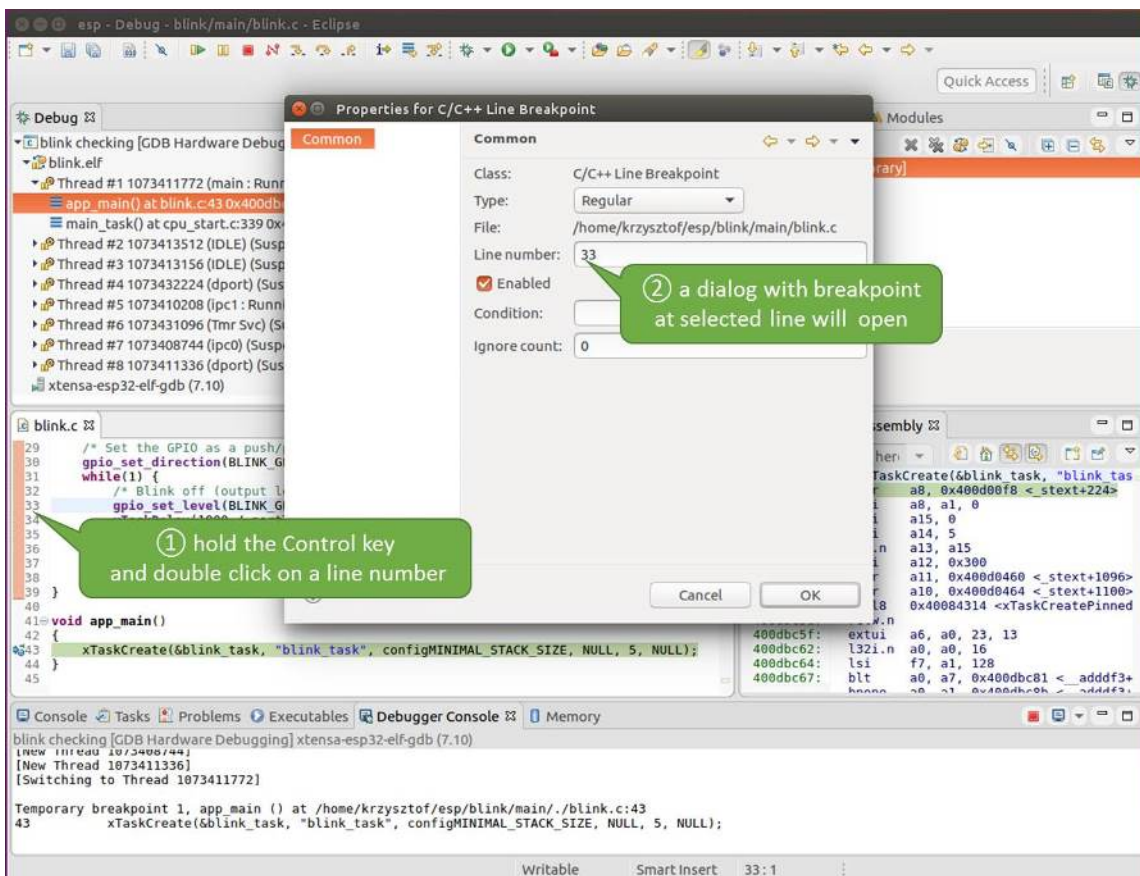
图 45: 设置断点
