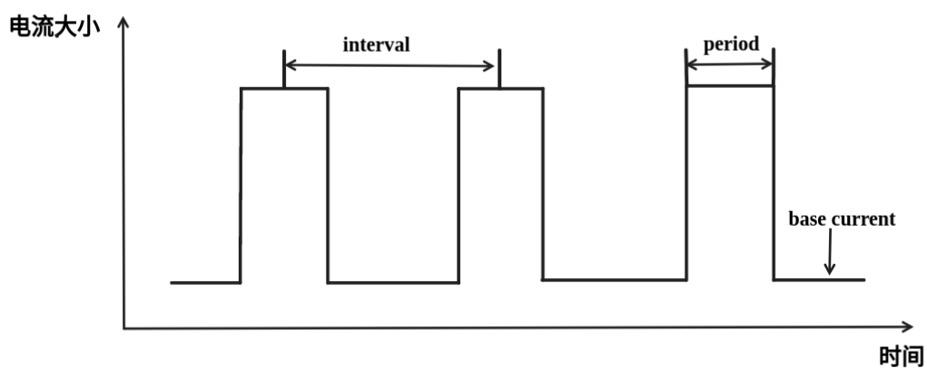
图 85: 理想情况下 Wi-Fi 场景低功耗模式电流图
