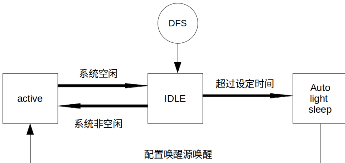
图 41: Auto Light-sleep 模式工作流程图
