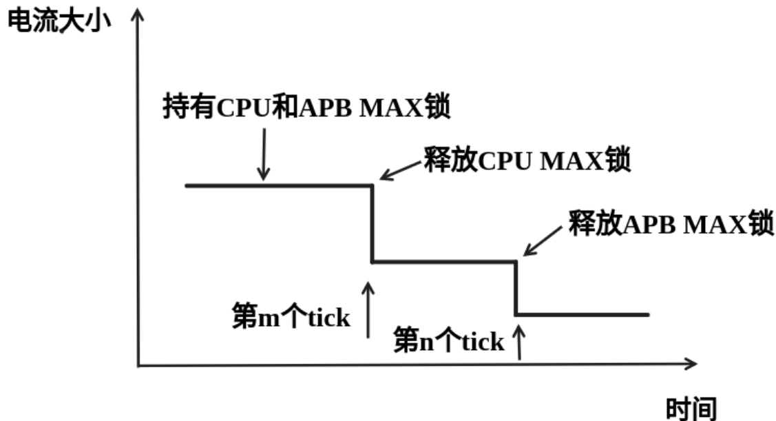
图 40: 理想 DFS 机制调频电流图
