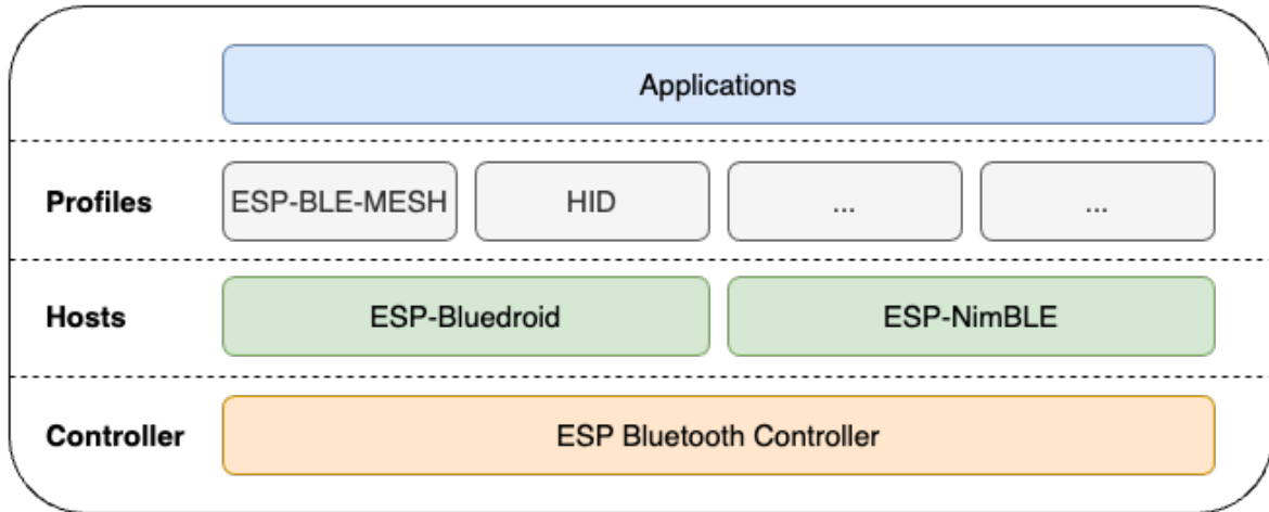
图 2: ESP32-H2 蓝牙协议栈架构
