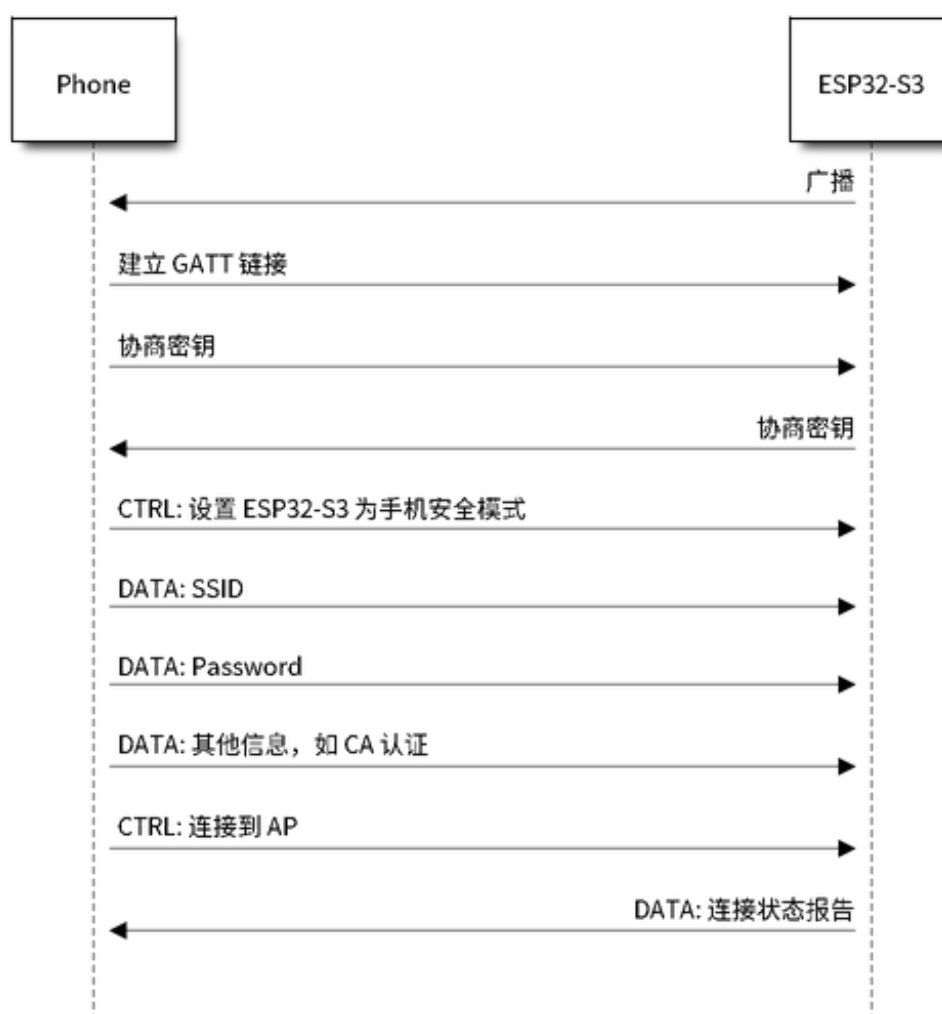
图 15: BluFi Flow Chart
