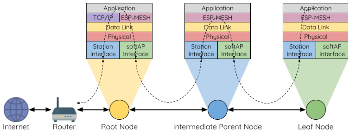
图 36: ESP-WIFI-MESH 双向数据流
