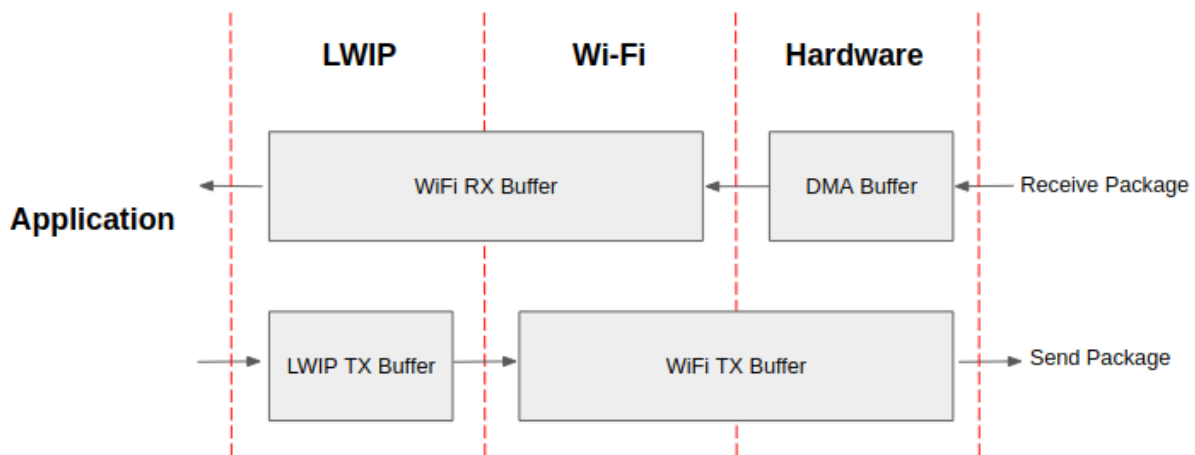
图 63: ESP32-S3 数据路径
