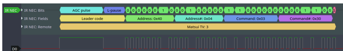
图 17: IR NEC Frame
