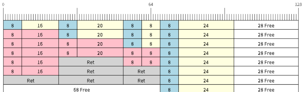
图 38: 在不可分割和可分割环形 buffer 中检索/返回数据项
