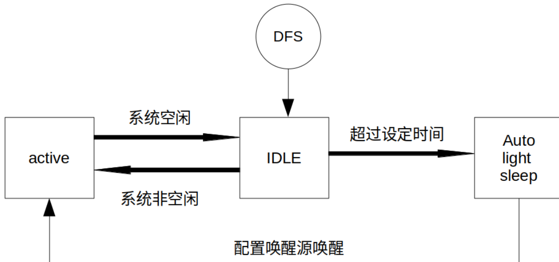
图 70: Auto Light-sleep 模式工作流程图
