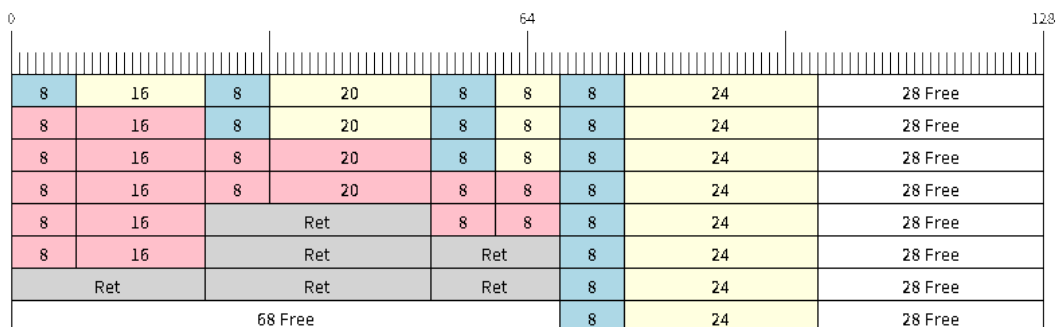
图 45: 在不可分割和可分割环形 buffer 中检索/返回数据项
