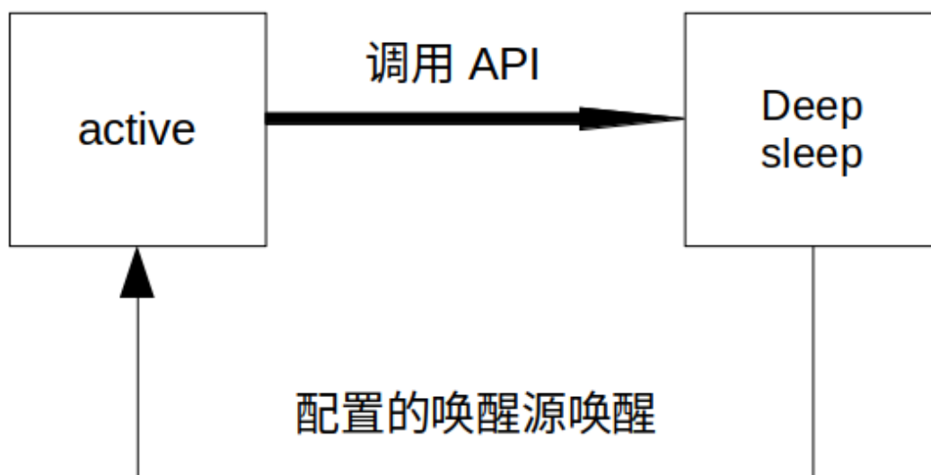
图 72: Deep-sleep 模式工作流程图
