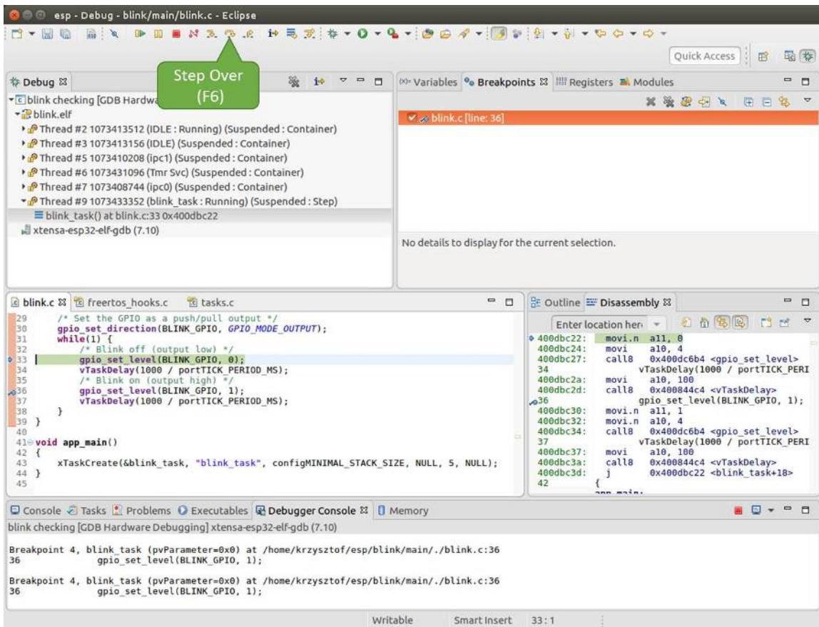
图 23: 使用“Step Over (F6)”单步执行代码
