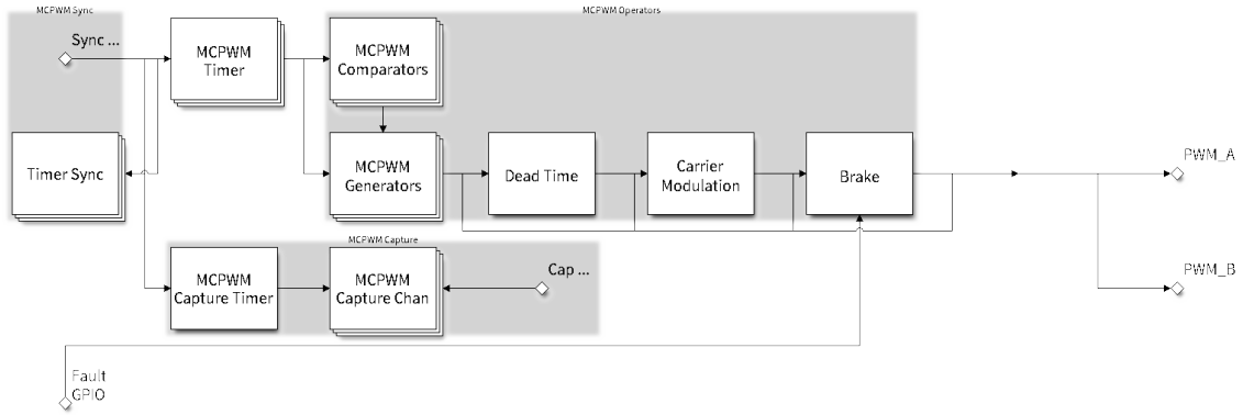
图 14: MCPWM 概述
