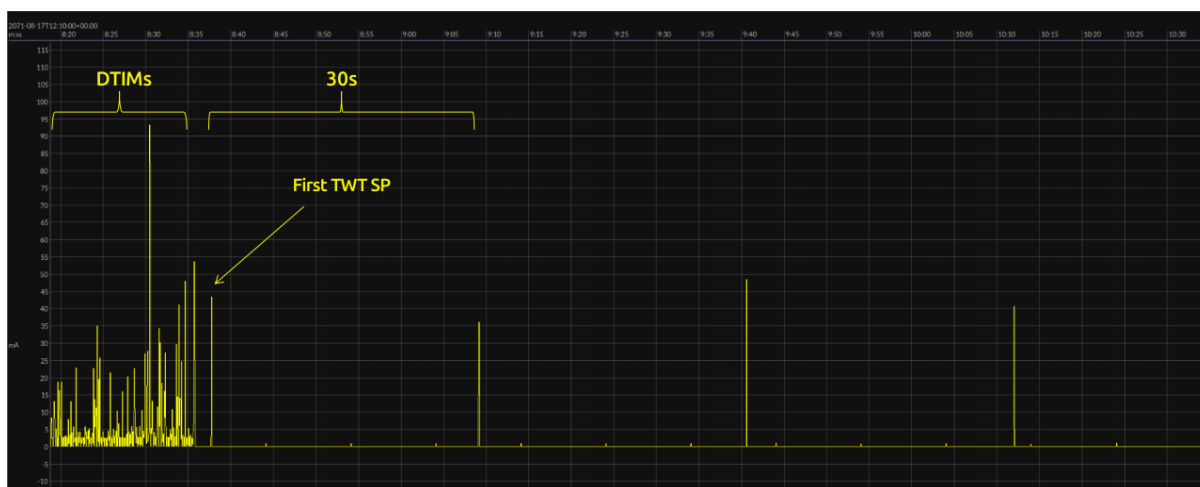
图 97: 更改参数后的 DTIM 与 iTWT 模式下的电流图
