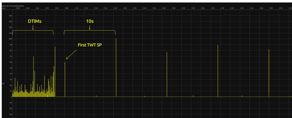
图 96: DTIM 与 iTWT 模式下的电流图
