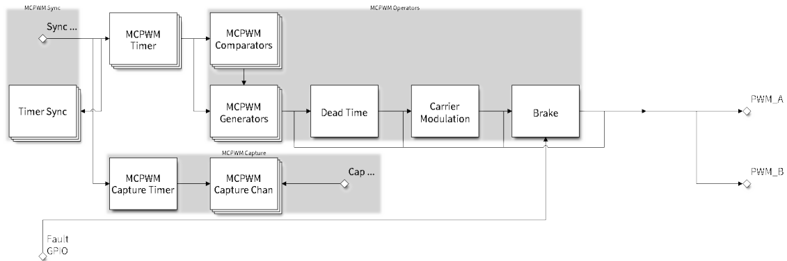
图 17: MCPWM 概述
