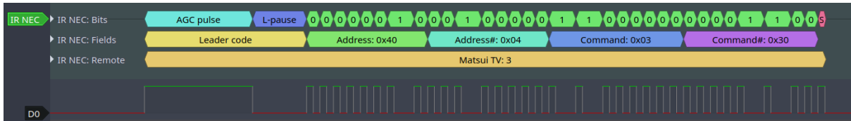
图 23: 红外 NEC 帧
