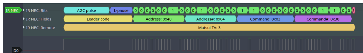
图 22: 红外 NEC 帧
