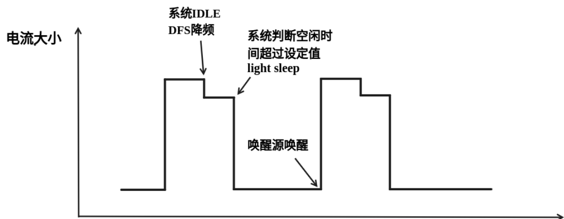
图 30: Auto Light-sleep 模式模式理想电流图
