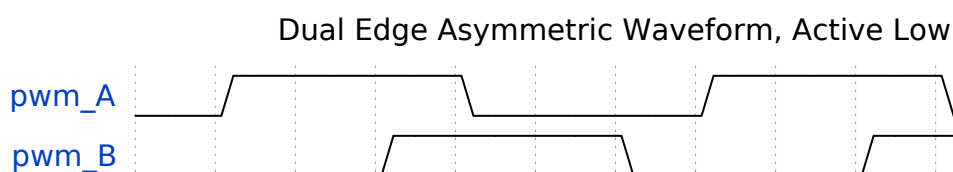
双沿不对称波形 - 低电平有效
