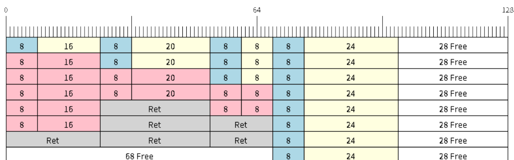
图 30: 在不可分割和可分割环形 buffer 中检索/返回数据项
