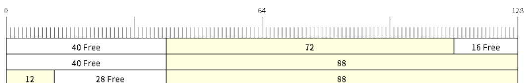
图 29: 在字节 buffer 中绕回
