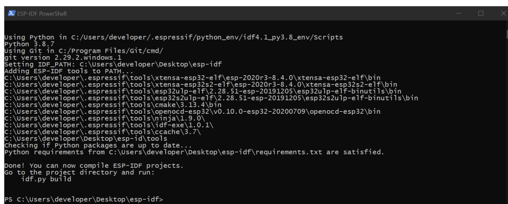
图 2: ESP-IDF PowerShell
