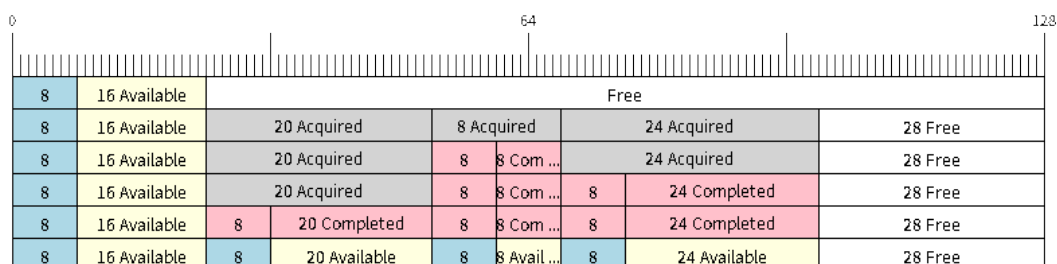
图 26: 在不可分割环形 buffer 中 SendAcquire/SendComplete 数据项
