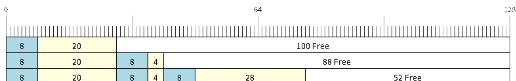
图 24: 向不可分割或可分割的环形 buffer 发送数据项
