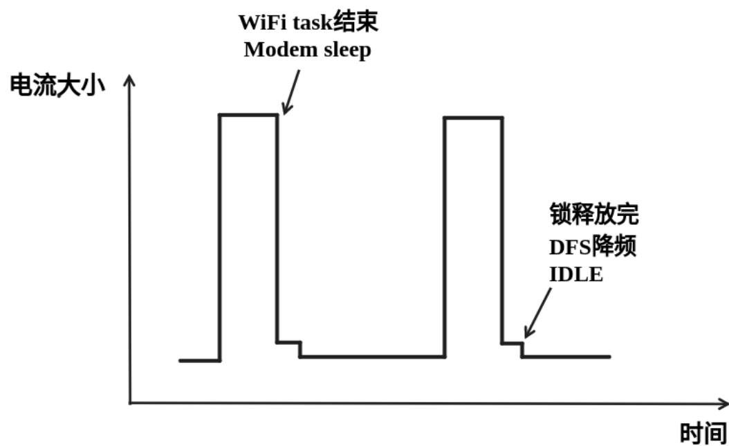
图 61: DFS+Modem sleep 模式理想电流图
