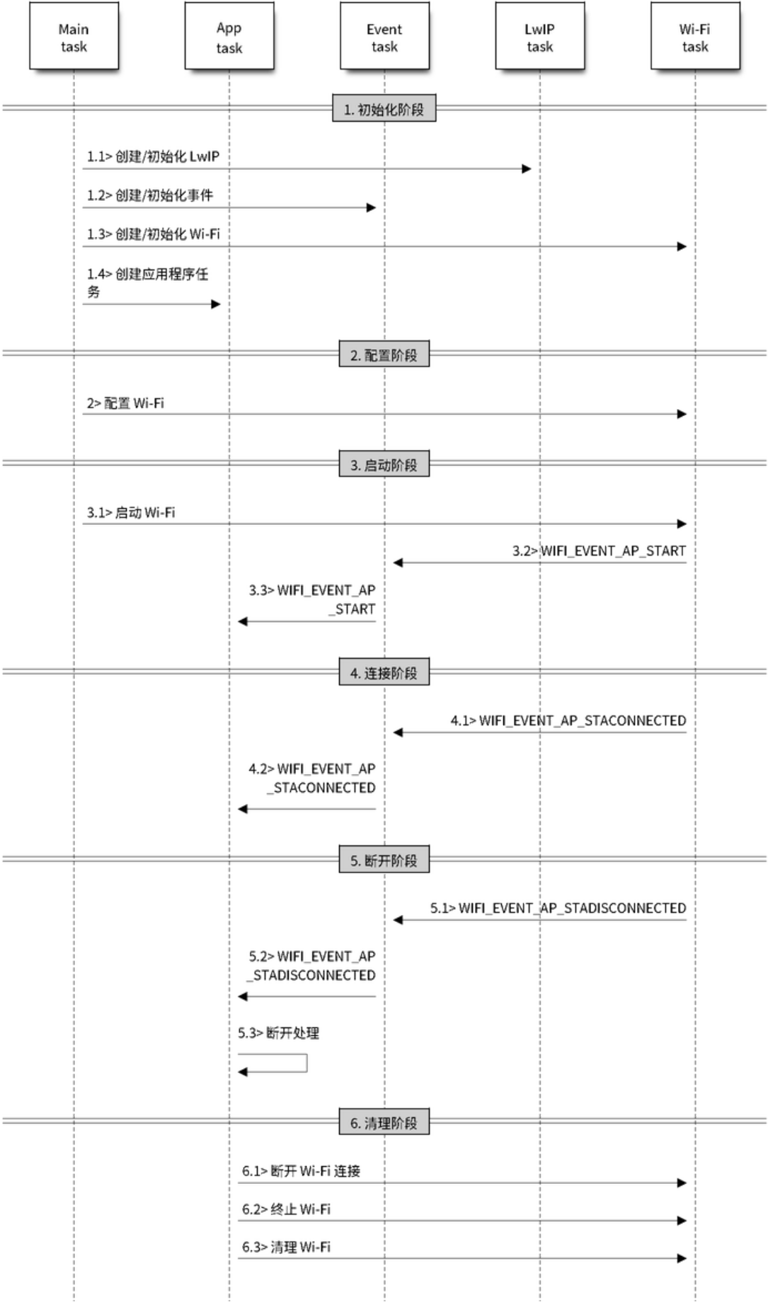
图 32: AP 模式下 Wi-Fi 事件场景示例
