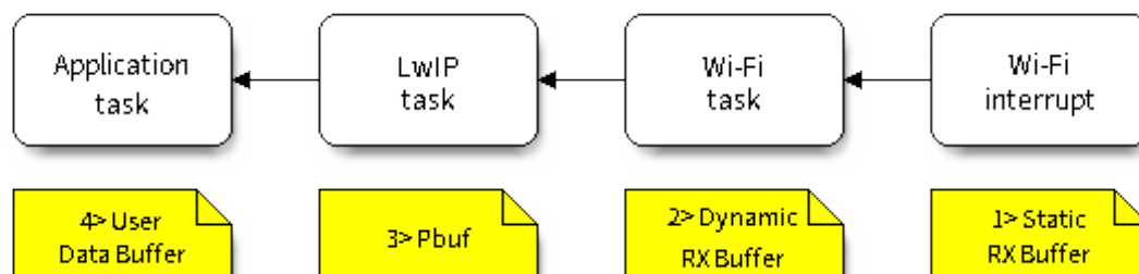
图 39: 接收数据缓冲区分配
