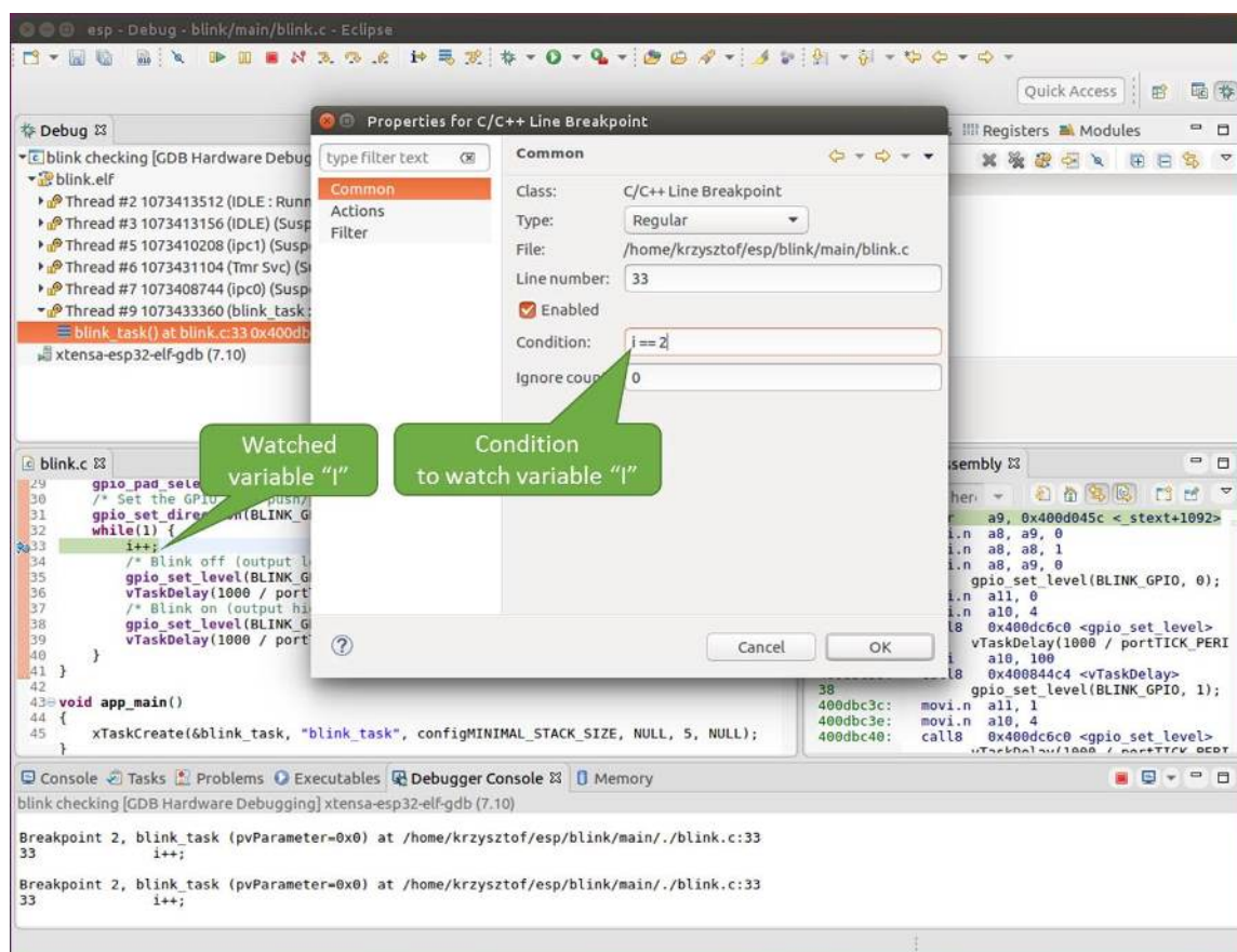
图 28: 设置条件断点
