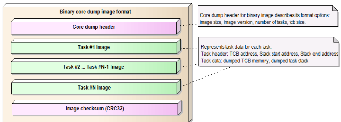
图 6: 核心转储二进制镜像文件格式
