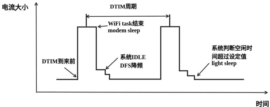
图 63: modem+auto light-sleep 模式理想电流图
