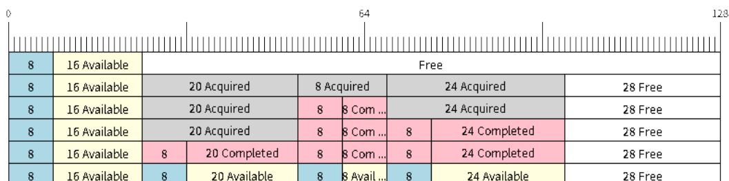
图 16: 在不可分割环形 buffer 中 SendAcquire/SendComplete 数据项
