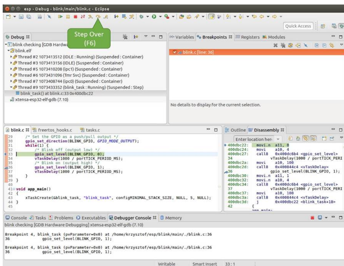
图 23: 使用“Step Over (F6)”单步执行代码
