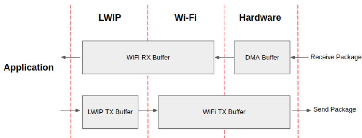
图 37: ESP32-C2 数据路径
