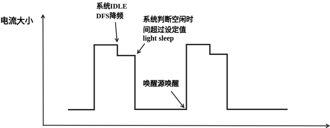
图 52: Auto Light-sleep 模式模式理想电流图
