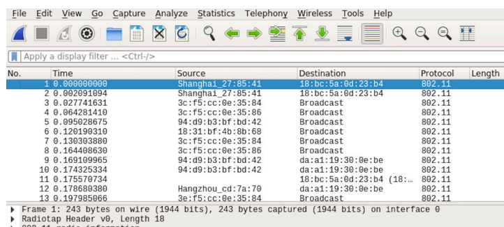
图 48: 开始或继续包的捕捉
