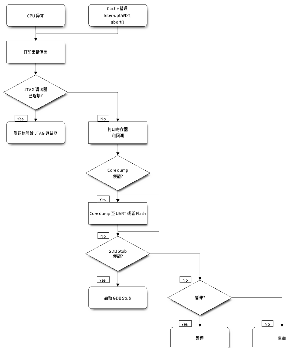
图 11: 紧急处理程序流程图 (点击放大)
