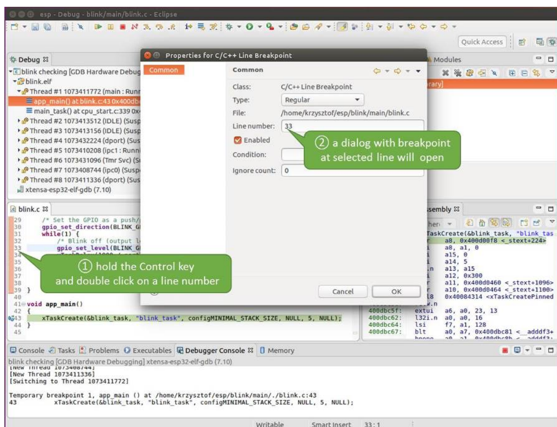
图 20: 设置断点
