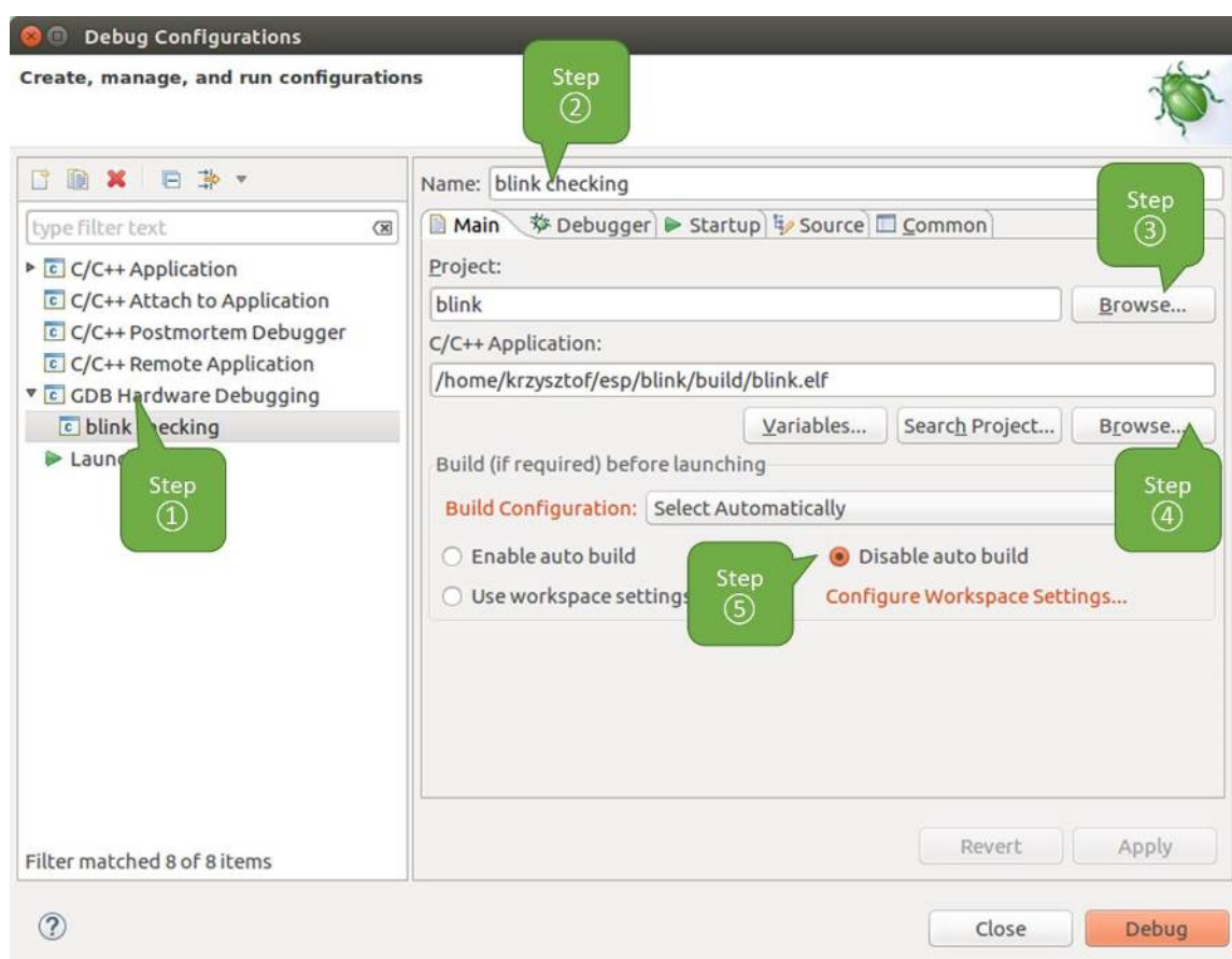
图 13: GDB 硬件调试的配置 - Main 选项卡
