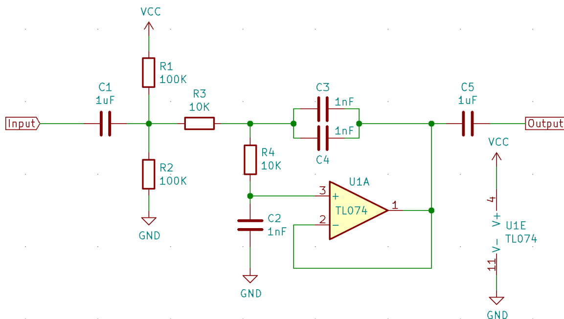
图 22: Sallen-Key 拓扑低通滤波器
