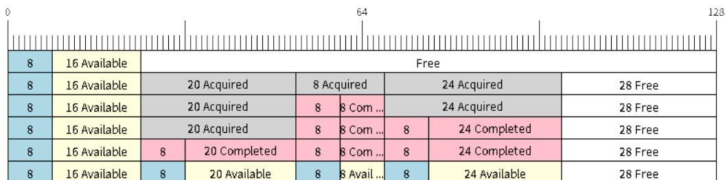
图 34: 在不可分割环形 buffer 中 SendAcquire/SendComplete 数据项
