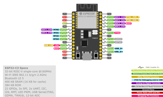
图 8: ESP32-C3-DevKitC-02 管脚布局 (点击放大)
