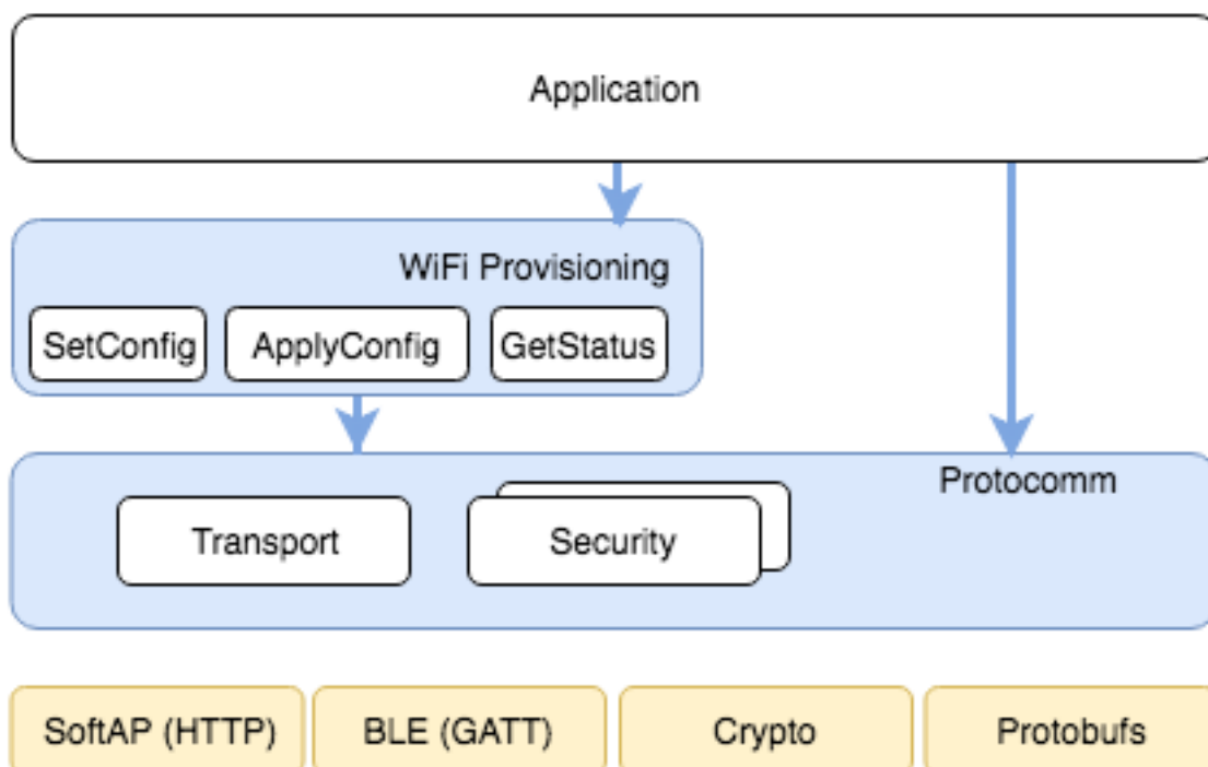
图 36: 统一配网架构
