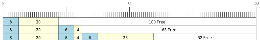
图 39: 向不可分割或可分割的环形 buffer 发送数据项
