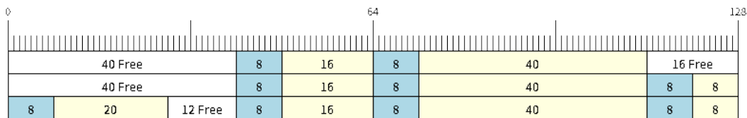
图 43: 在可分割 buffer 中绕回
