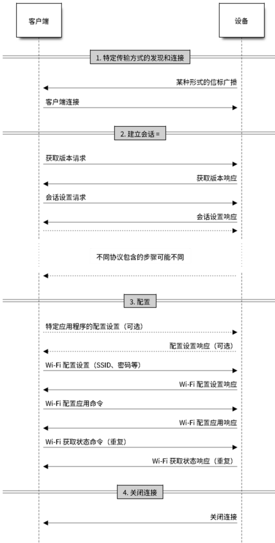
图 35: 配网过程示例
