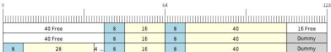
图 42: 在不可分割 buffer 中绕回
