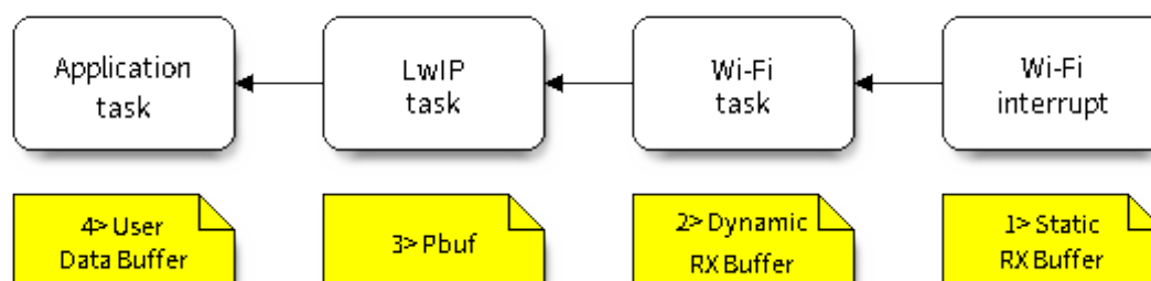
图 41: 接收数据缓冲区分配
