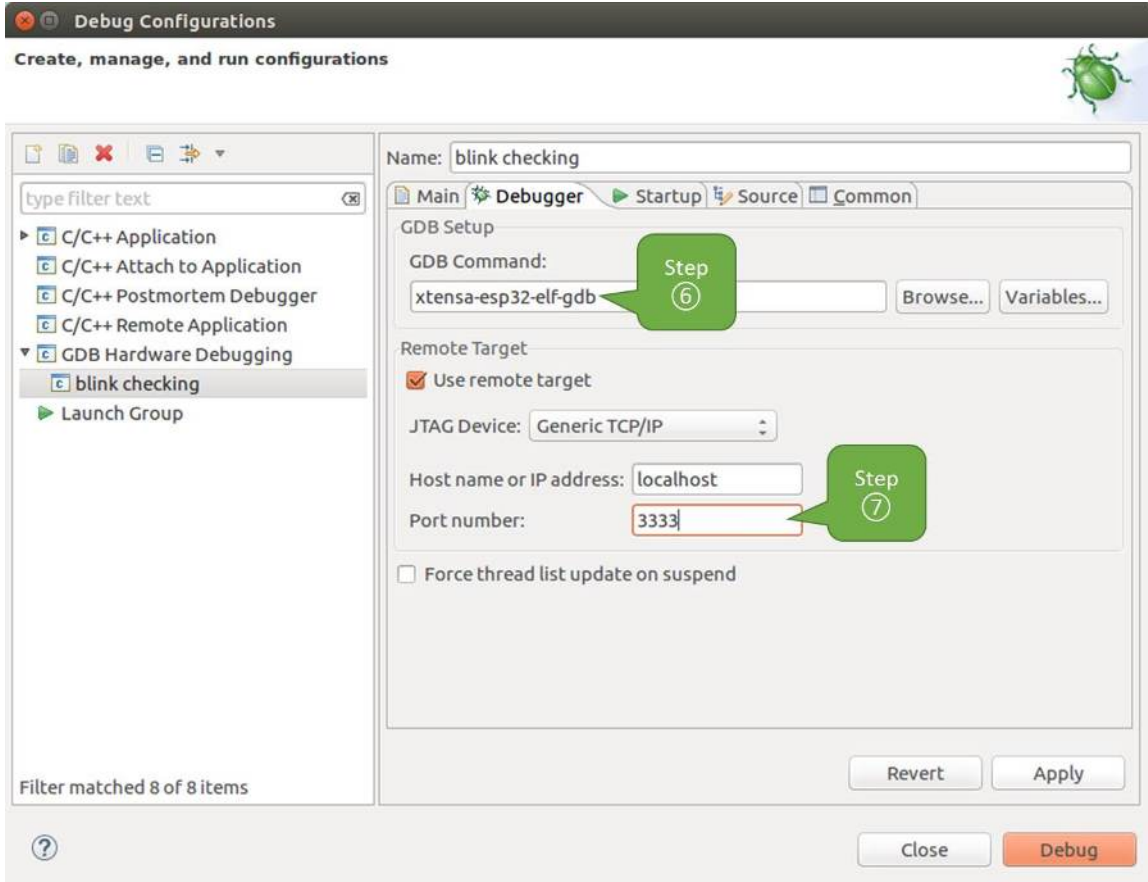
图 16: GDB 硬件调试的配置 - Debugger 选项卡
