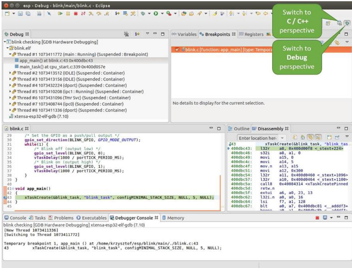
图 18: Eclipse 中的调试视图
