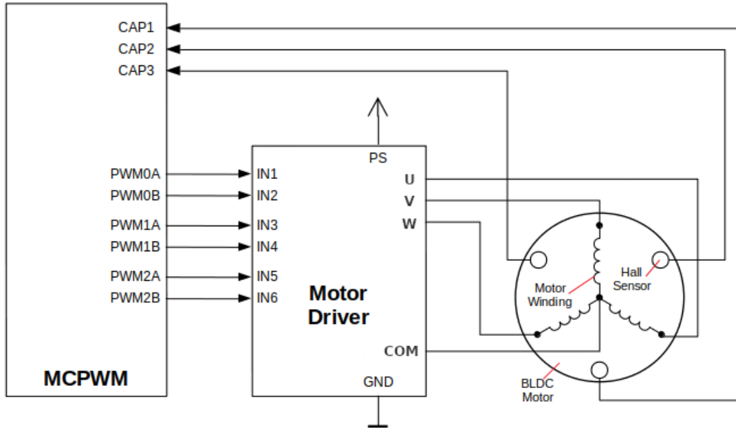
图 17: 带霍尔传感器的 MCPWM 无刷直流电机
