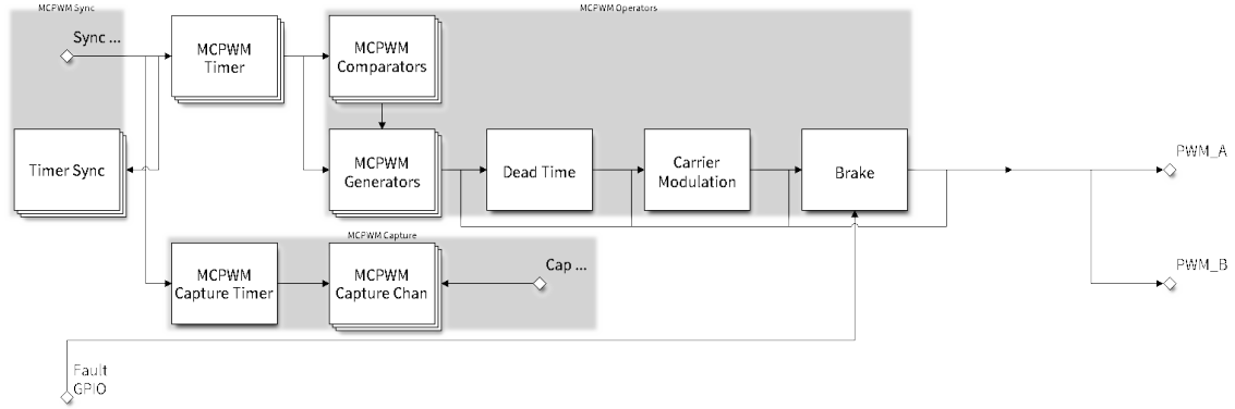
图 16: MCPWM 概述
