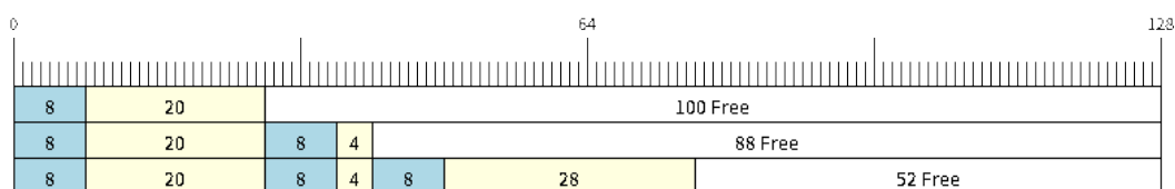
图 40: 向不可分割或可分割的环形 buffer 发送数据项
