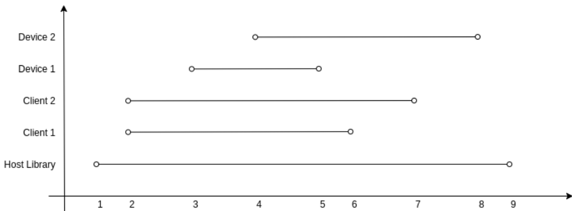
图 34: USB 主机库典型生命周期
