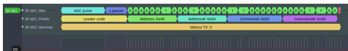
图 24: 红外 NEC 帧
