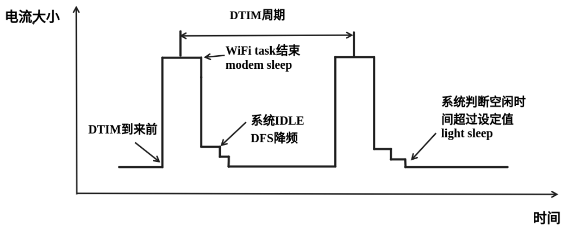
图 92: modem + auto light-sleep 模式理想电流图
