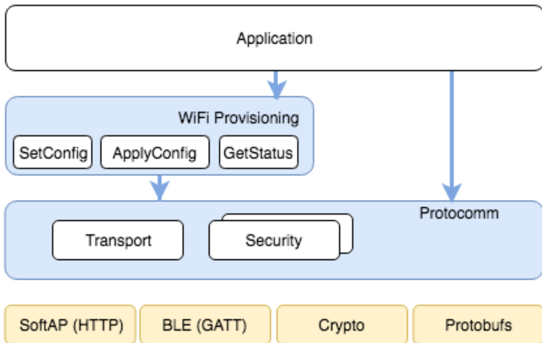
图 37: 统一配网架构
