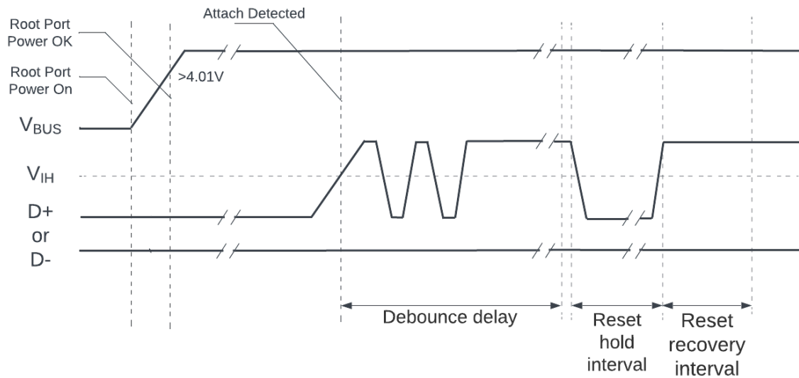
图 35: USB 根集线器上电和连接事件时序
