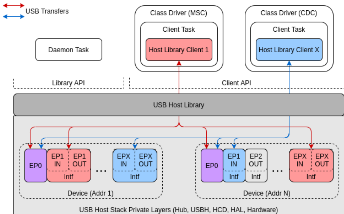
图 33: USB 主机功能涉及的关键实体
