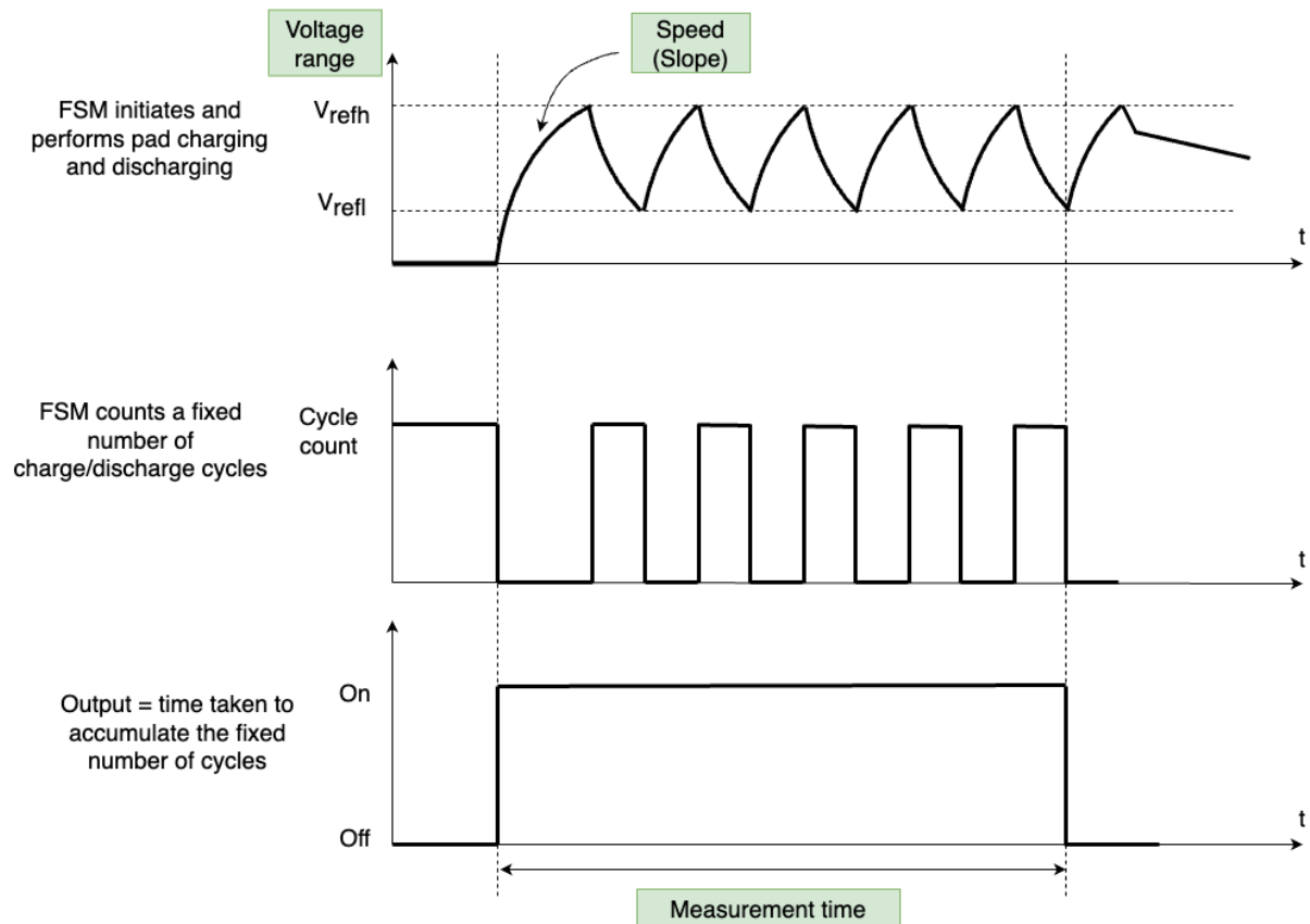
图 26: 触摸传感器 - 测量参数之间的关系
