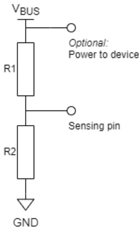
图 32: 用于 VBUS 监测的简易分压器
