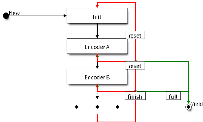
图 23: RMT 编码器链
