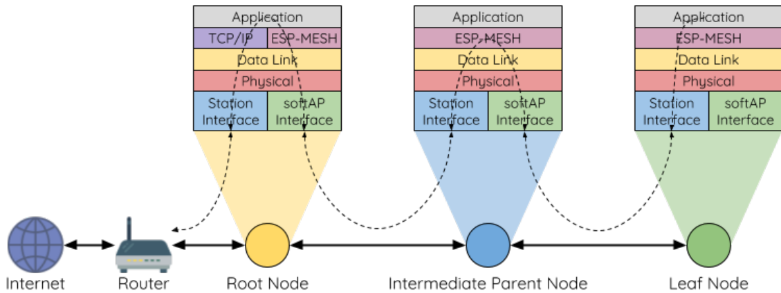
图 60: ESP-WIFI-MESH 双向数据流
