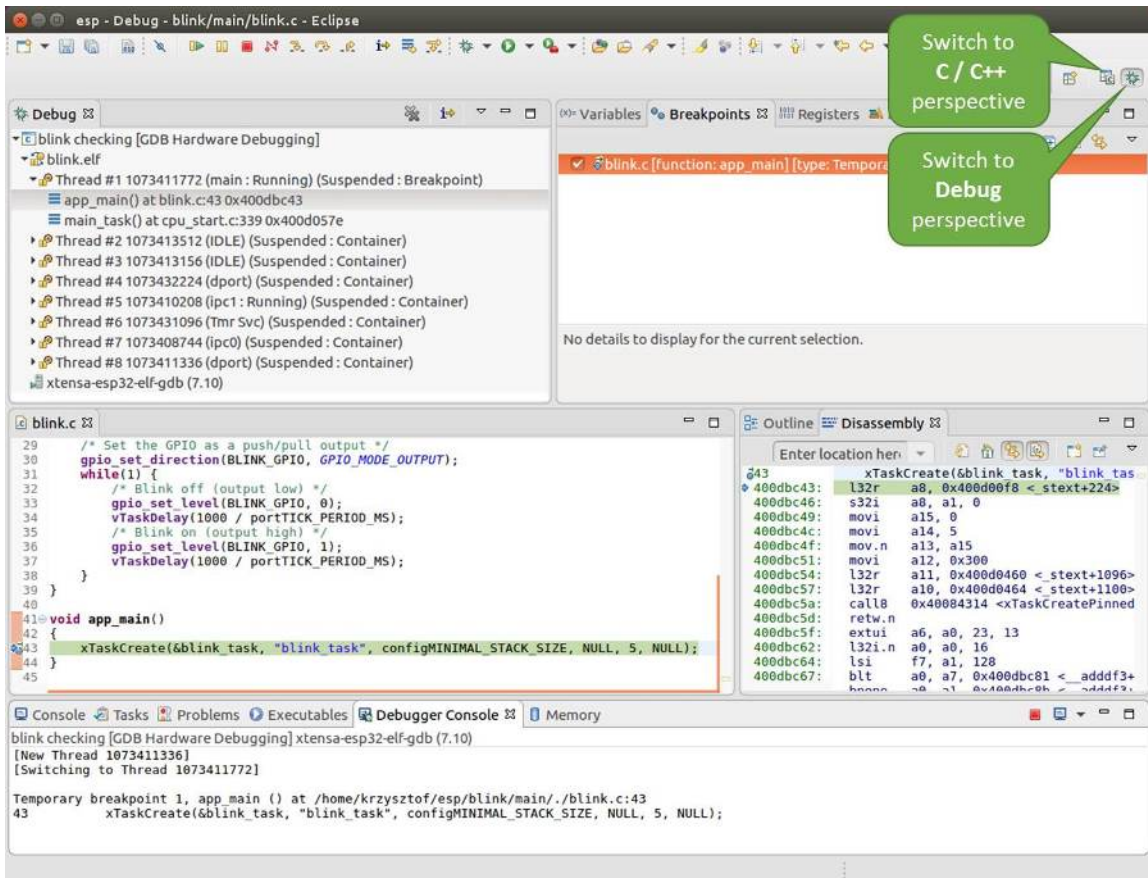
图 67: Eclipse 中的调试视图
