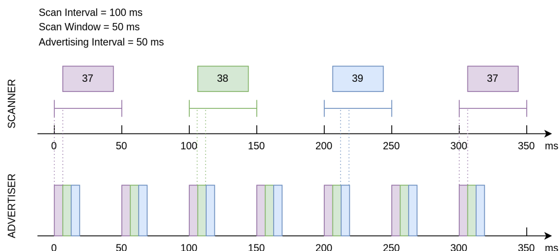
图 16: 广播与扫描时序示意图
