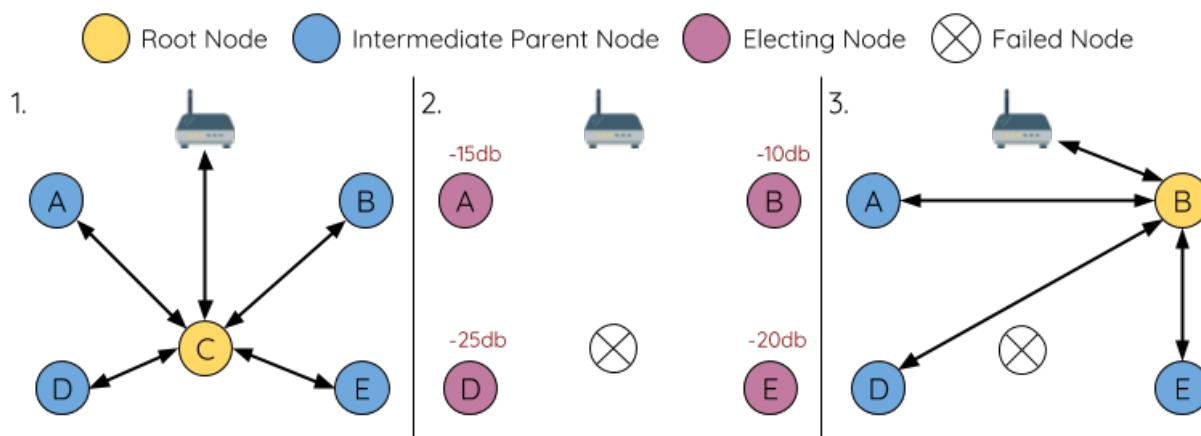
图 57: 根节点故障的自修复示意
