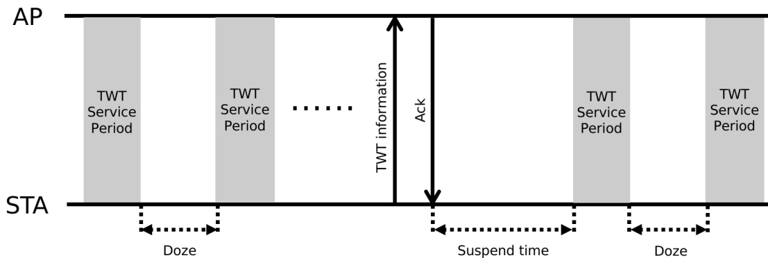
图 114: Individual TWT 协商暂停/恢复过程示例
