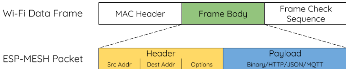
图 58: ESP-WIFI-MESH 数据包
