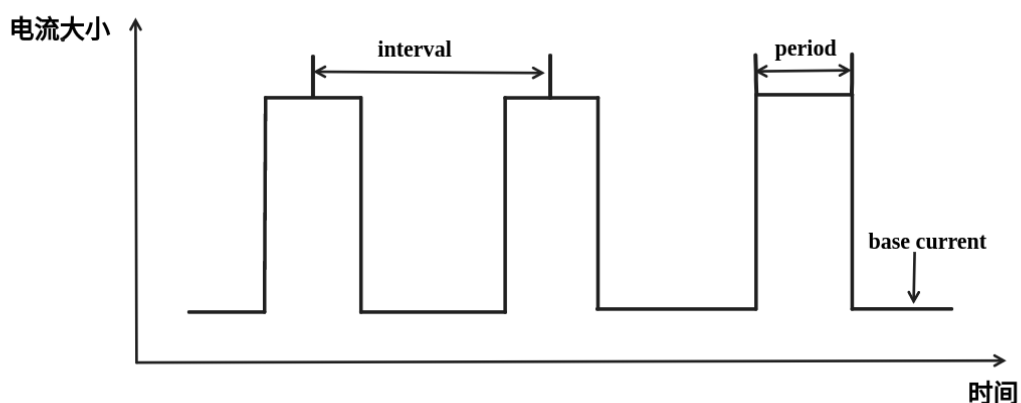
图 106: 理想情况下 Wi-Fi 场景低功耗模式电流图
