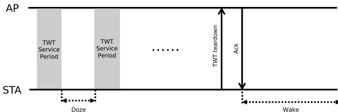
图 115: Individual TWT 协商终止过程示例
