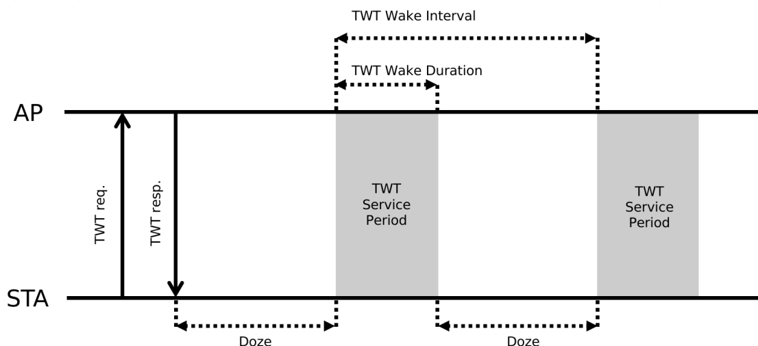
图 113: Individual TWT 协商建立过程示例
