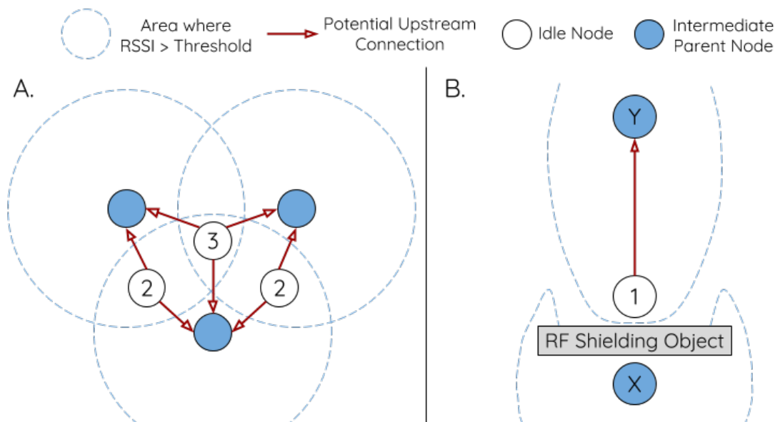
图 49: RSSI 阈值的影响
