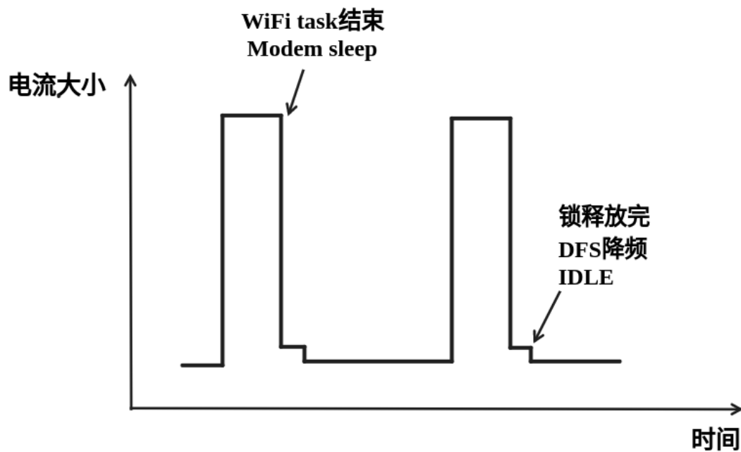
图 110: DFS + Modem sleep 模式理想电流图
