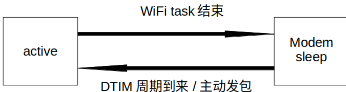
图 107: Modem sleep 工作流程图
