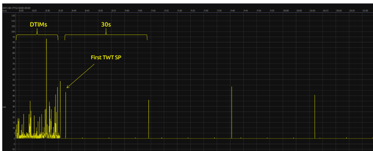
图 117: 更改参数后的 DTIM 与 iTWT 模式下的电流图
