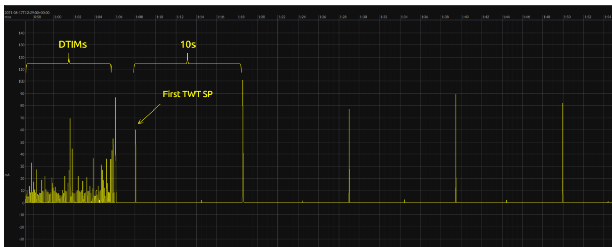
图 116: DTIM 与 iTWT 模式下的电流图
