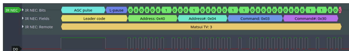
图 19: 红外 NEC 帧
